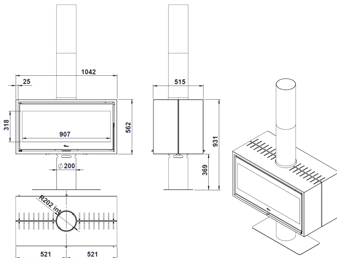
Figura nº4 - Dimensões em mm do aparelho Verona 1001
