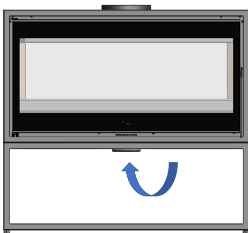
Figura nº10 - Condução do ar para a câmara de combustão Verona 1003
