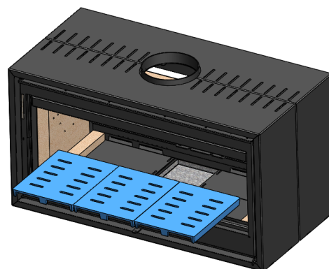
Figura nº17 - Extraímos a grelhas de ferro fundido
