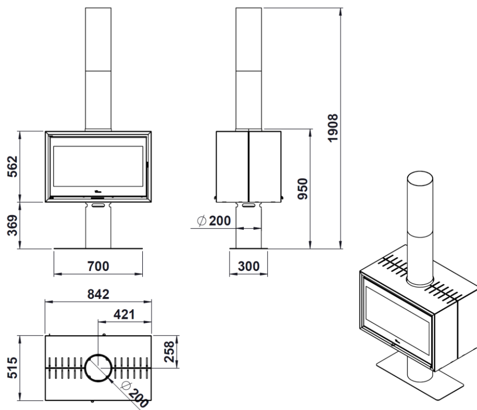
Figura nº2 - Dimensões em mm do aparelho Verona 801
