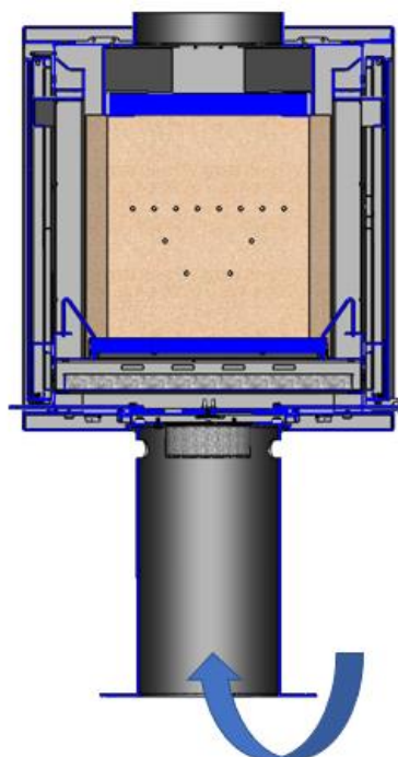
Figura nº9 - Condução do ar para a câmara de combustão Verona 801-1001
