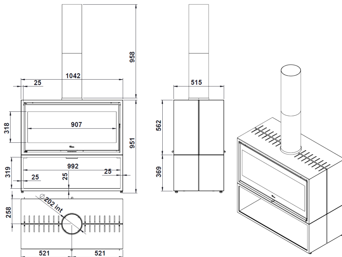
Figura nº5 - Dimensões em mm do aparelho Verona 1003
