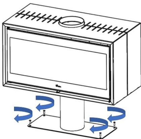
Figura nº7 - Fixação do Verona 801-1001 ao solo
