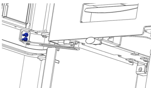
Figura nº21 - Passo 3. Desmontar parafusos do suporte da porta
