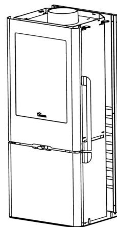
Figura nº26 - Passo 4. Montar dupla traseira
