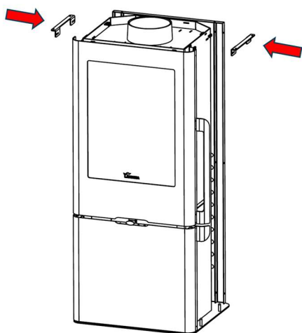
Figura nº28 - Passo 6. Montar suportes dos laterais de pedra serpentina
