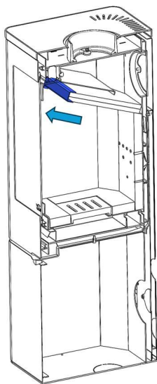
Figura nº15 - Extrair reforço
