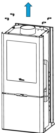
Figura nº27 - Passo 5. Desmontar suportes dos laterais de aço
