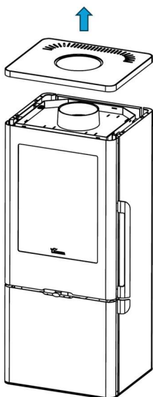
Figura nº23 - Passo 1. Desmontar tampa superior
