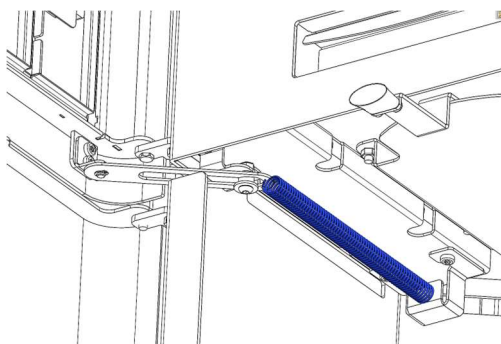
Figura nº19 - Passo 1. Desmontar mola
