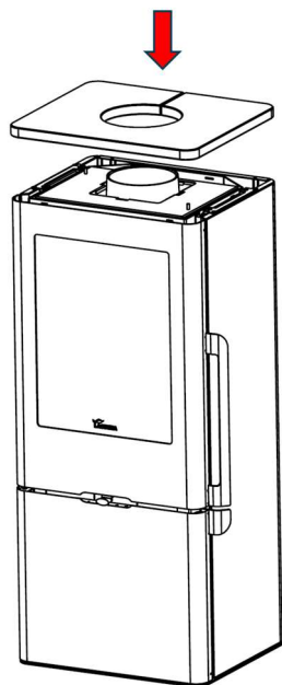
Figura nº32 - Passo 10. Colocar a tampa de pedra serpentina
