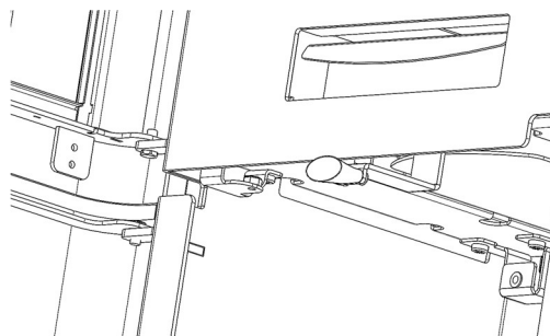
Figura nº22 - Passo 4. Retirar mecanismo
