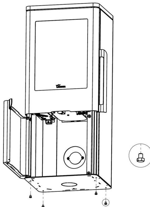
Figura nº18 - Instalação dos pés de nivelamento
