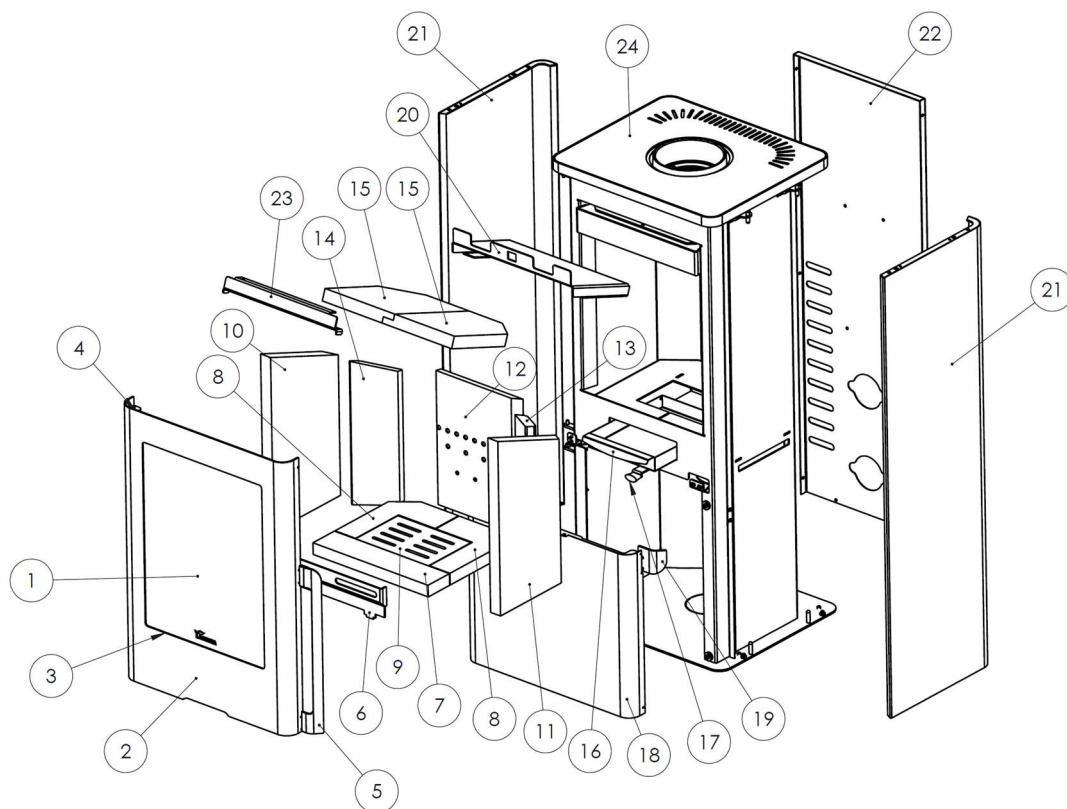
Figura nº33 - Explosão de peças VELA
