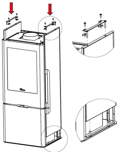
Figura nº31 - Passo 9. Colocar os laterais de pedra serpentina e fixá-los com os suportes
