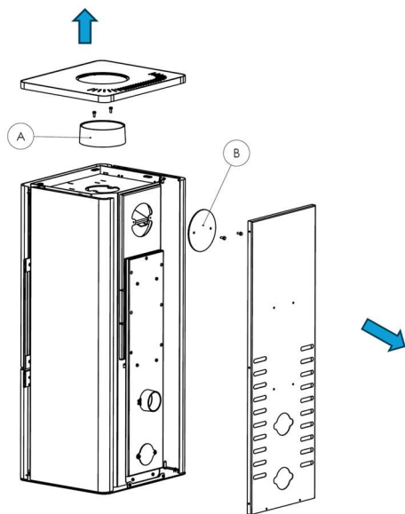
Figura nº5 - Trocar os componentes (A) e (B) para saída de fumos posterior
