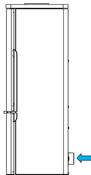
Figura nº7 - OPÇÃO 2 Condução de ar para a câmara de combustão
