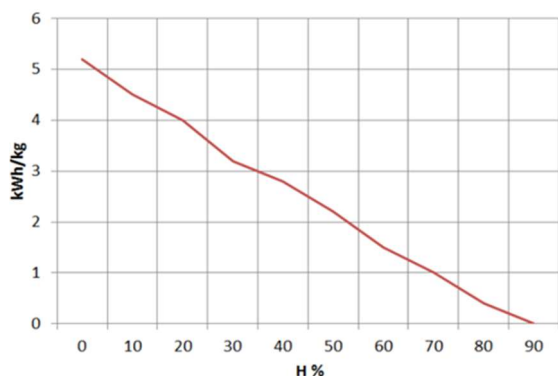
Figura n°12 - Relação entre humidade e poder calorífico da lenha.
