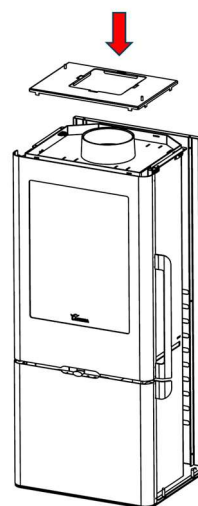
Figura nº30 - Passo 8. Montar suporte da tampa de pedra serpentina
