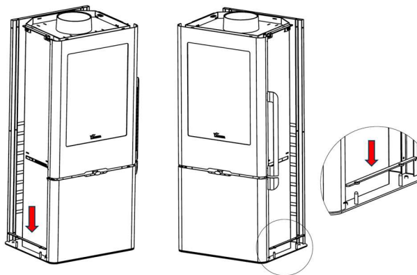
Figura nº29 - Passo 7. Montar calços dos laterais de pedra serpentina
