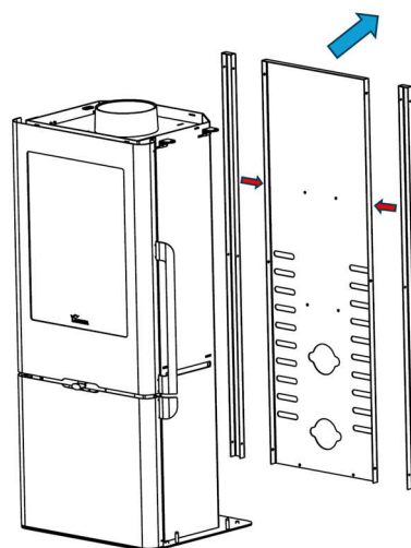
Figura nº25 - Passo 3. Desmontar dupla traseira e montar peças adicionais
