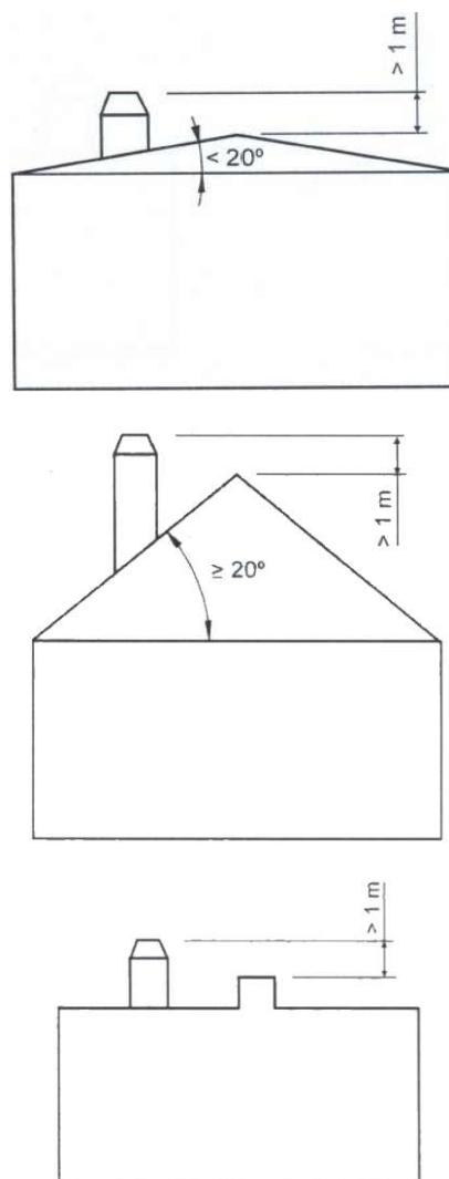
Figura nº9 - Distâncias desde o acabamento até à cumeeira do telhado
