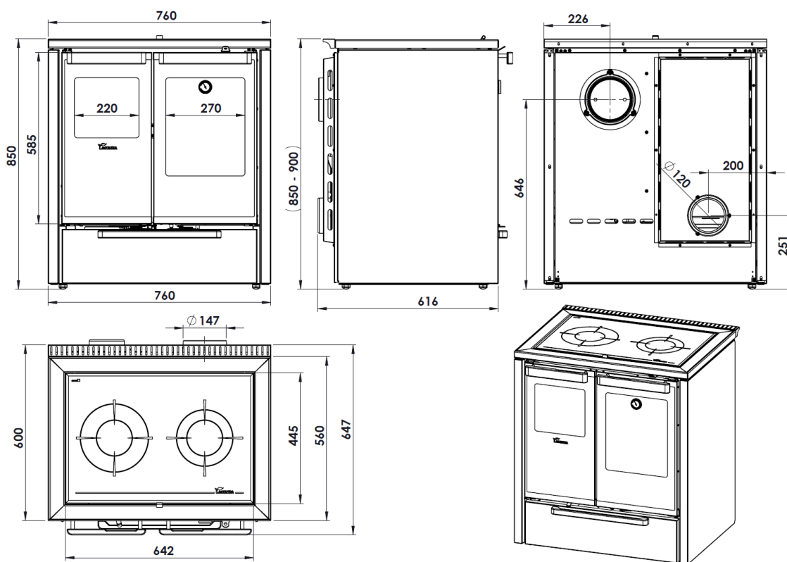
Figura nº2 - Dimensões em mm do aparelho TERRA 5T Super V
