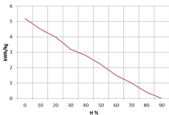
Figura nº15 - Relação entre umidade e poder calorífico da lenha.
