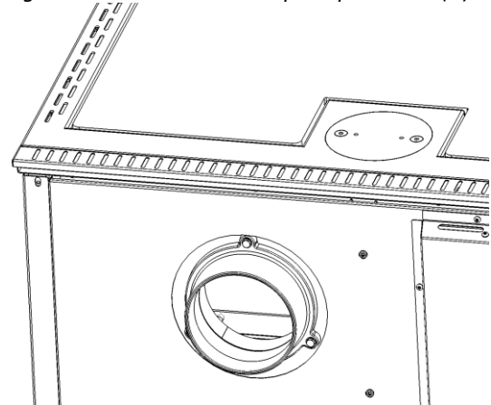
Figura nº10 - Situação final, adequada para uma saída de fumos superior.
