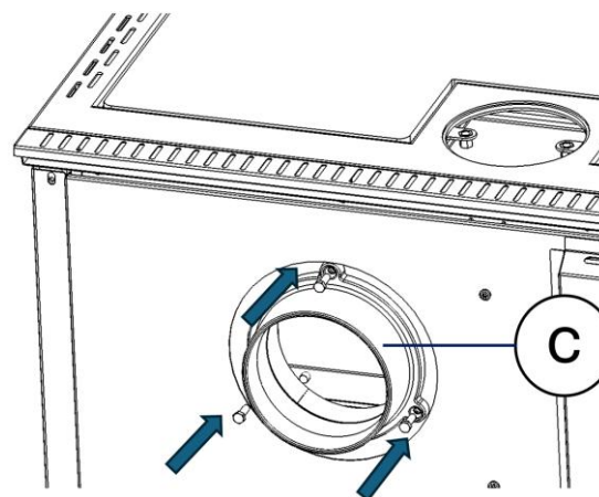
Figura nº8 - Colocamos a saída de fumo traseira (C).
