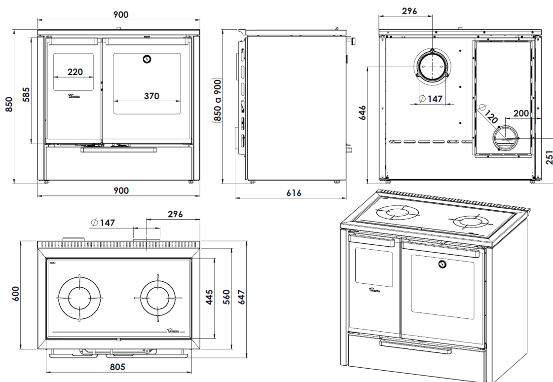
Figura nº4 - Dimensões em mm do aparelho TERRA 7T Super V
