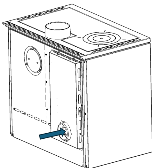
Figura nº11 - Conduta de ar para a câmara de combustão.
