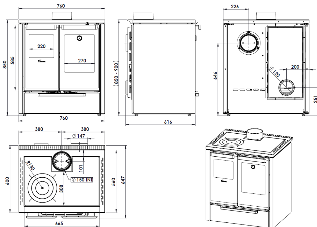
Figura nº1 - Dimensões em mm do aparelho TERRA 5T saída de fumos SUP CEN inox
