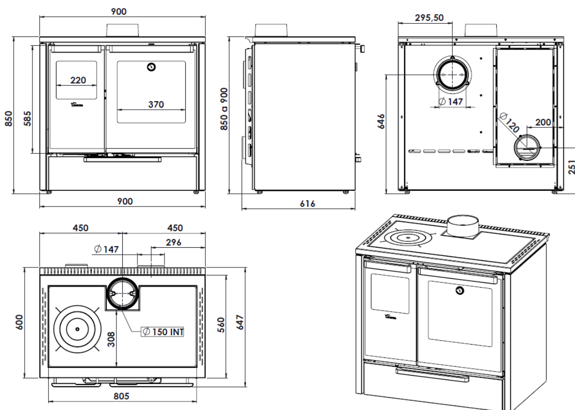
Figura nº3 - Dimensões em mm do aparelho TERRA 7T S-SUP CEN inox
