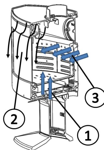
Figura nº16 - Entradas de ar de combustão
