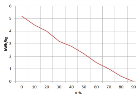
Figura nº14 - Relação entre humidade e poder calorífico da lenha.
