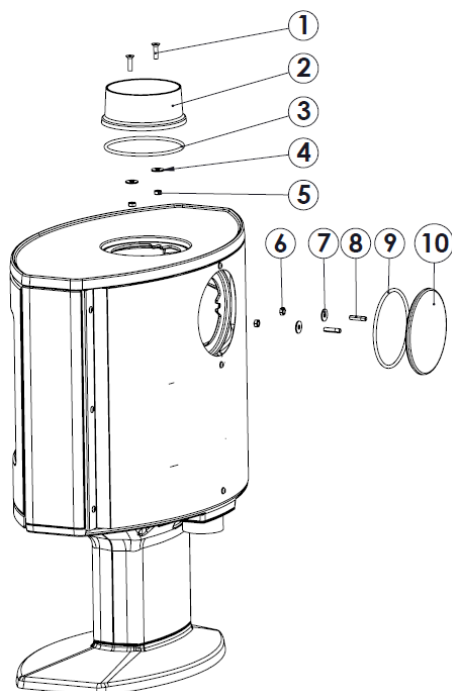
Figura nº8 - Desmontagem de tampa traseira e anel de ligação superior
