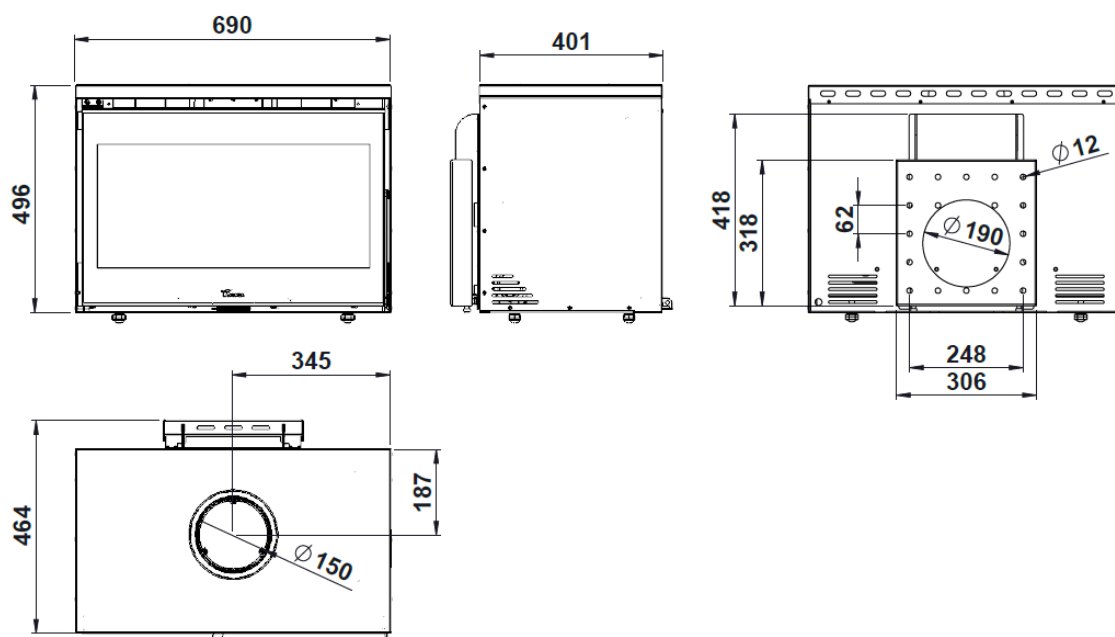
Figura n°3 - Dimensões em mm do aparelho PARIS 700 MURAL
