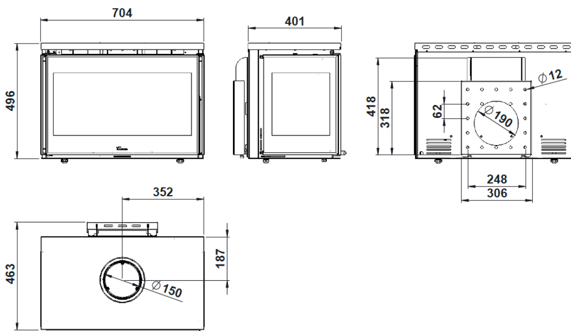
Figura n°4 - Dimensões em mm do aparelho PARIS 700 CLID MURAL
