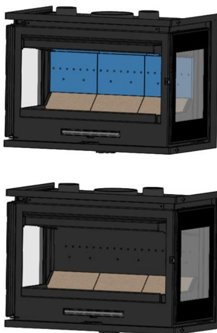
Figura nº22 - Desmontagem defletor
