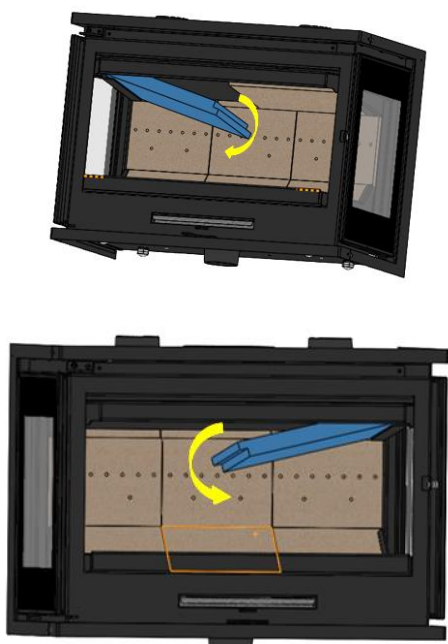
Figura nº22 - Desmontagem defletor
