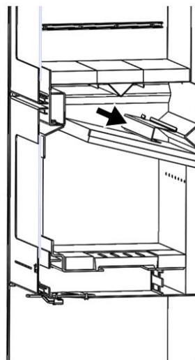
Figura nº13 - Reforço sobre os defletores de vermiculita
