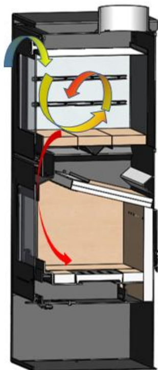
Figura nº8 - Esquema sistema de extração de vapores
