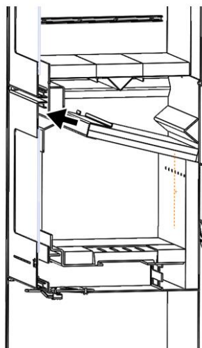
Figura nº11 - Primeiro movimento para soltar o reforço
