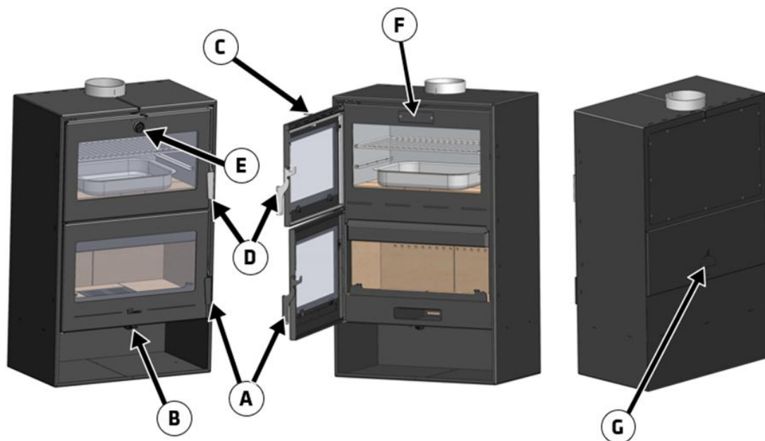
Figura nº7 - Elementos de funcionamento do aparelho
