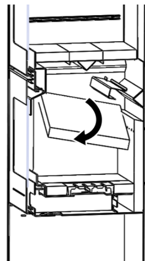
Figura nº14 - Extração dos defletores de vermiculita
