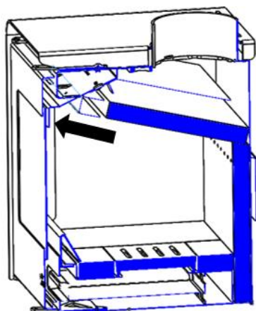
Figura nº10 - Primeiro movimento para soltar o reforço
