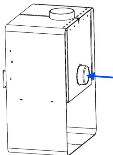
Figura nº3 - Condução de ar para câmara de combustão
