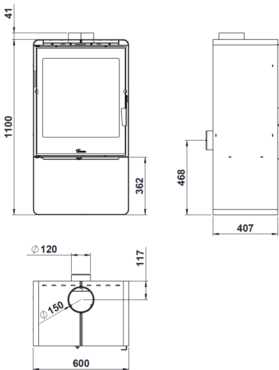
Figura nº1 - Dimensões em mm do aparelho Ocean/Atlantic 613
