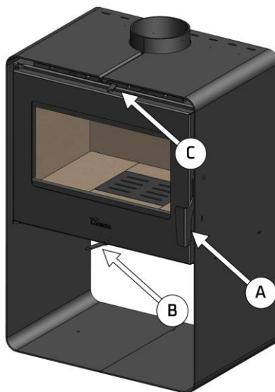
Figura nº9 - Elementos de funcionamento do aparelho
