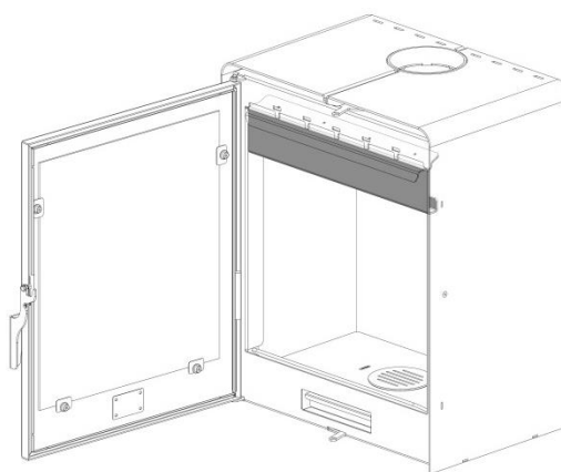
Figura nº7 - Acessório de ajuda para casos de retornos de fumos causados por uma instalação deficiente
