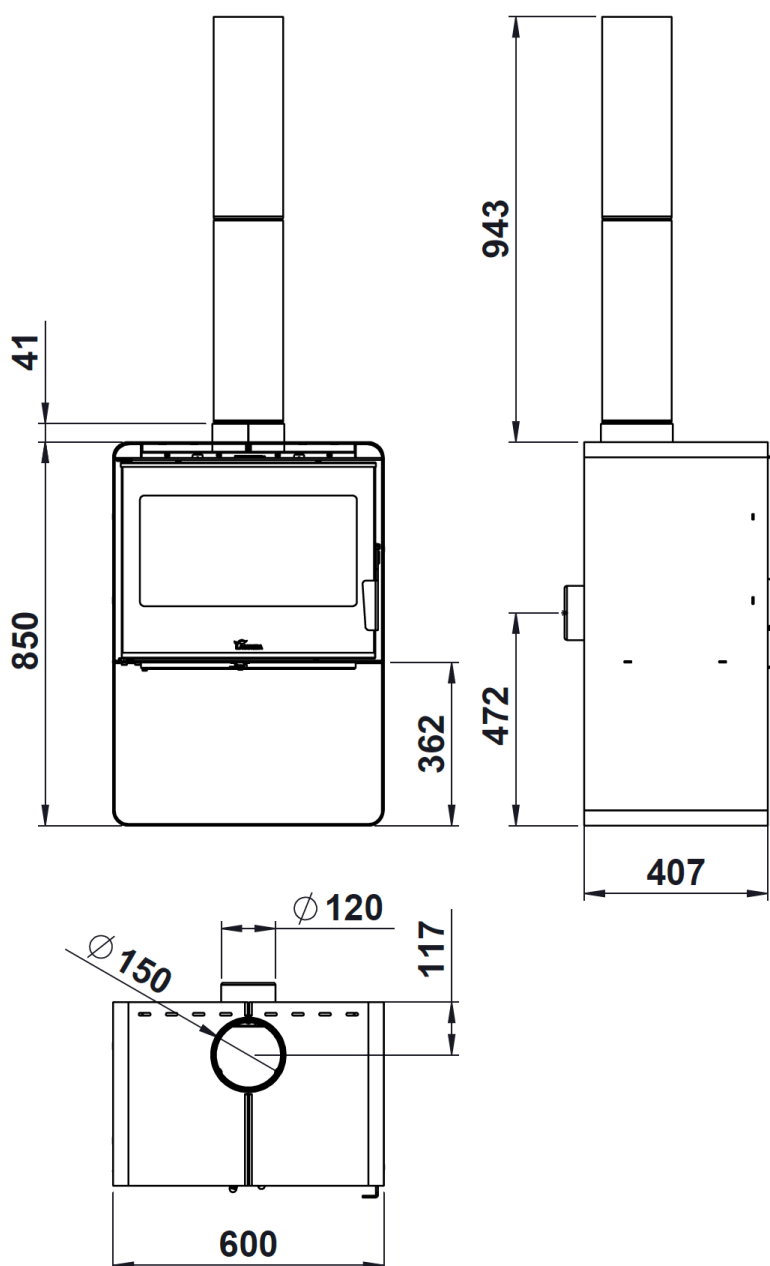
Figura nº1 - Dimensões em mm do aparelho Ocean/Atlantic 603
