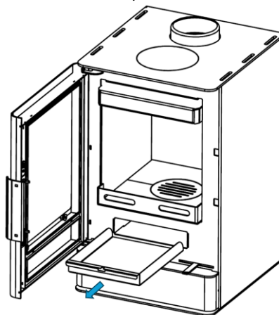
Figura nº11 - Extração do cinzeiro
