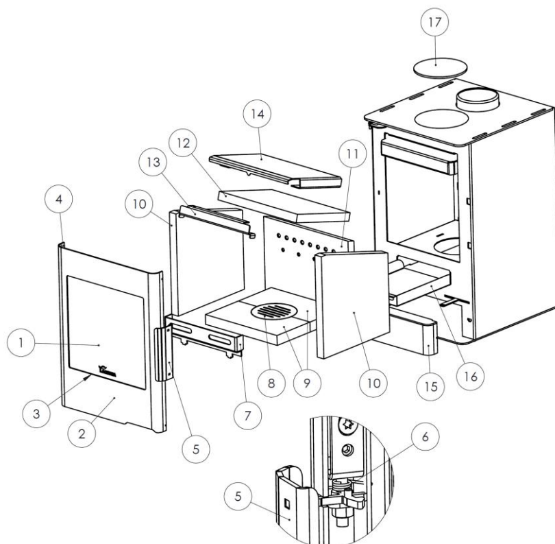
Figura nº23 - Explosão de peças VELA
