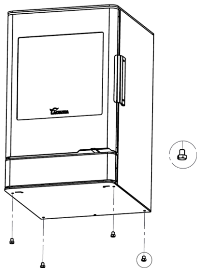
Figura nº16 - Instalação dos pés de nivelamento
