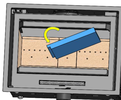
Figura nº23 - Desmontagem defletor
