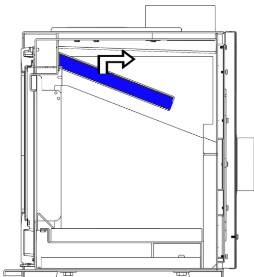
Figura nº16 - Desmontagem do deflector de aço
