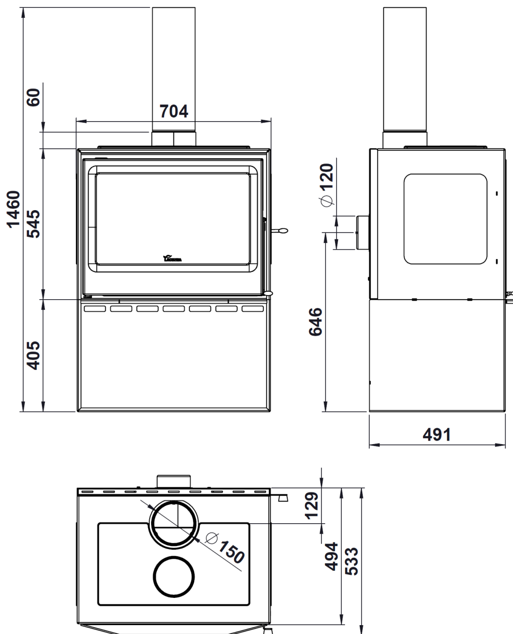
Figura nº2 - Dimensões em mm do aparelho MARTINA L
