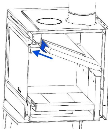
Figura nº14 - Retirar o reforço
