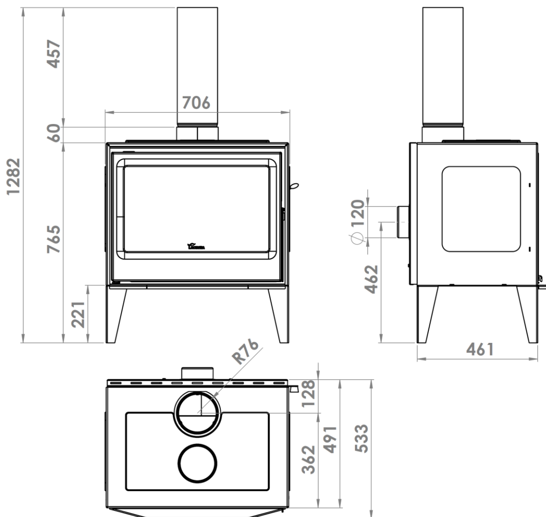
Figura nº1 - Dimensões em mm do aparelho MARTINA
