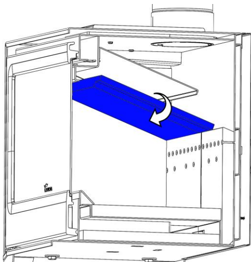
Figura nº15 - Remover a vermiculite
