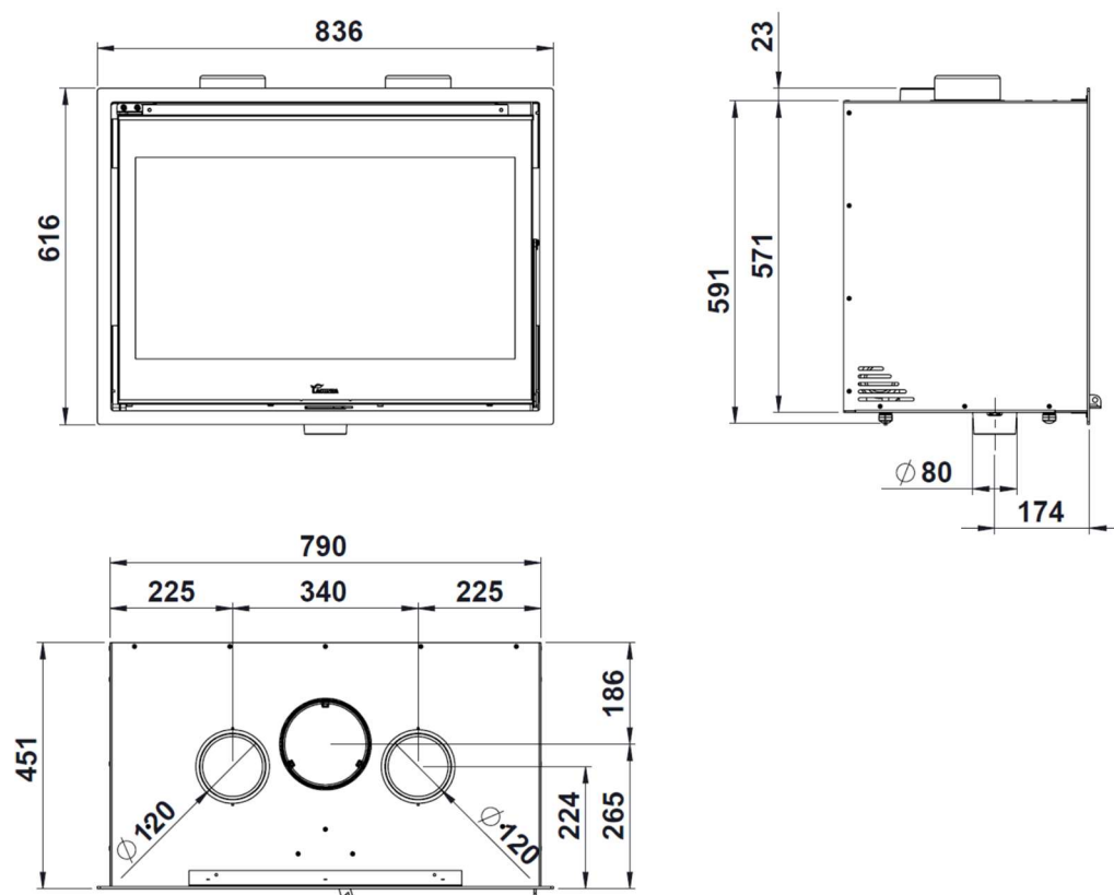
Figura nº2 - Dimensões em mm do aparelho LOIRE 800
