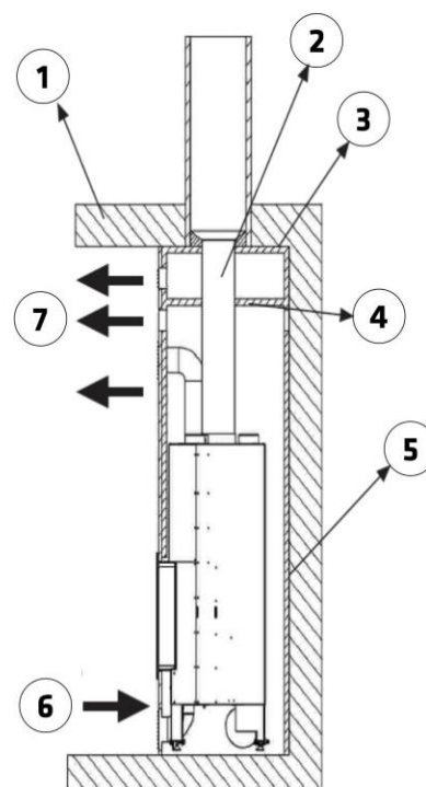
Figura nº7 - Esquema interior do fecho
