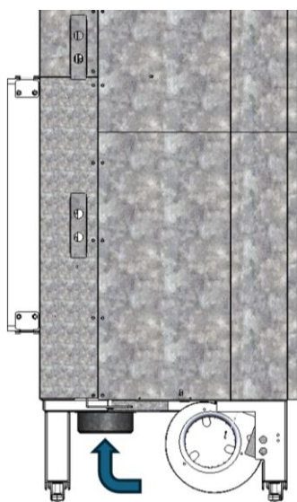
Figura nº9 - Conduatas de ar para a câmara de combustão
