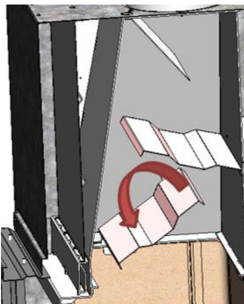
Figura nº33 - Desmontagem do defletor médio Itaca 80 eco
