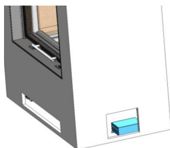
Figura nº19 - Posicionamento do módulo de potência em frente à grade de ventilação lateral
