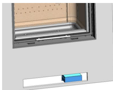
Figura nº18 - Posicionamento do módulo de potência em frente à grade de ventilação frontal
