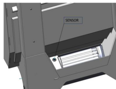
Figura nº20 - Posição da sonda de temperatura (SENSOR) na saída de ar da turbina
