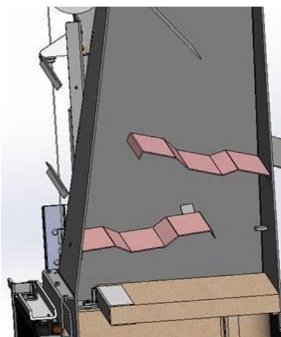
Figura nº26 - Posição atual dos defletores
