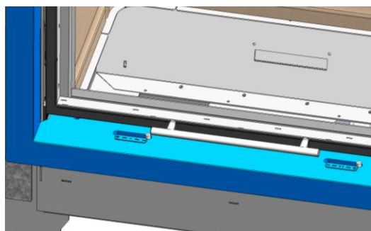
Figura nº47 - Quadro externo
