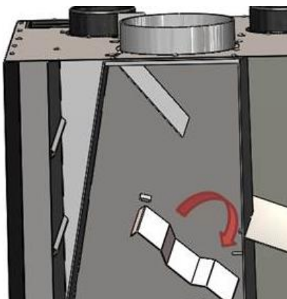
Figura nº33 - Desmontagem do defletor superior Itaca 80
