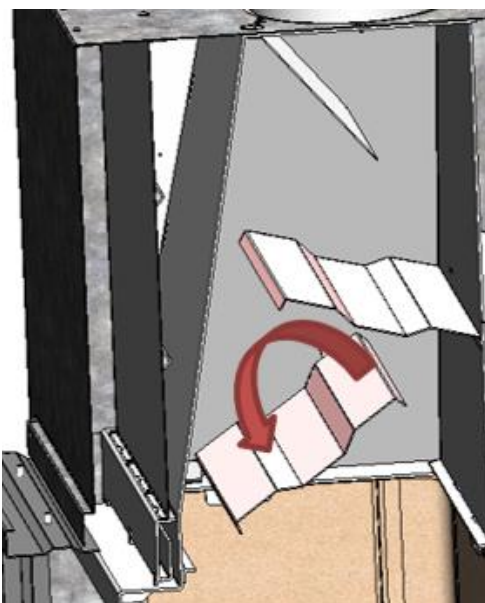
Figura nº32 - Desmontagem do defletor médio Itaca 80 eco
