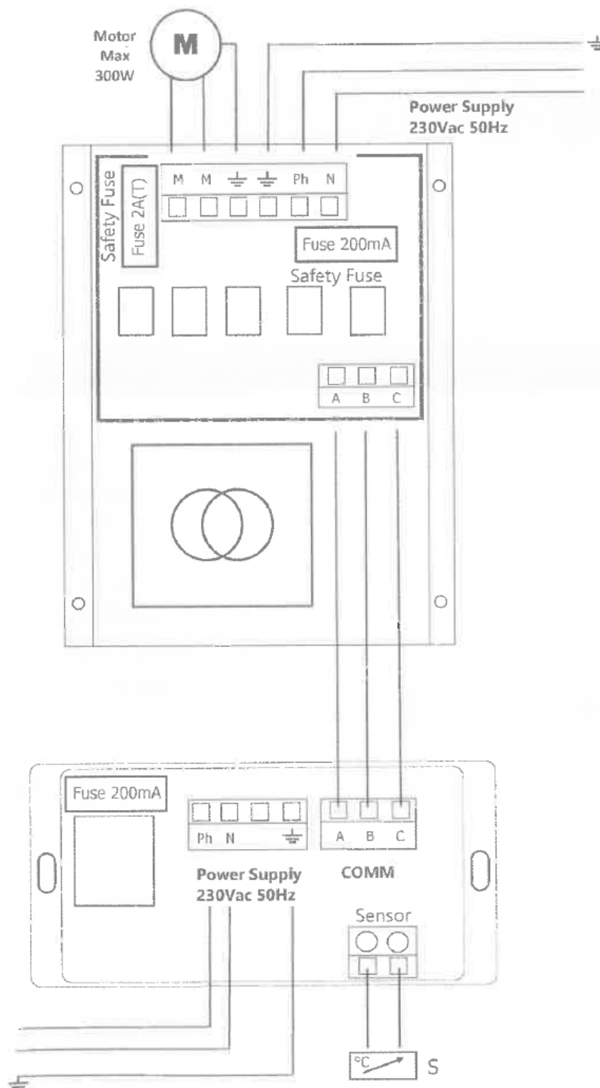
Figura nº17 - Conexões a serem feitas no controlador e no módulo de potência do Itaca eco C / V
