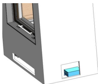
Figura nº20 - Posicionamento do módulo de potência em frente à grade de ventilação lateral
