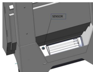
Figura nº21 - Posição da sonda de temperatura (SENSOR) na saída de ar da turbina
