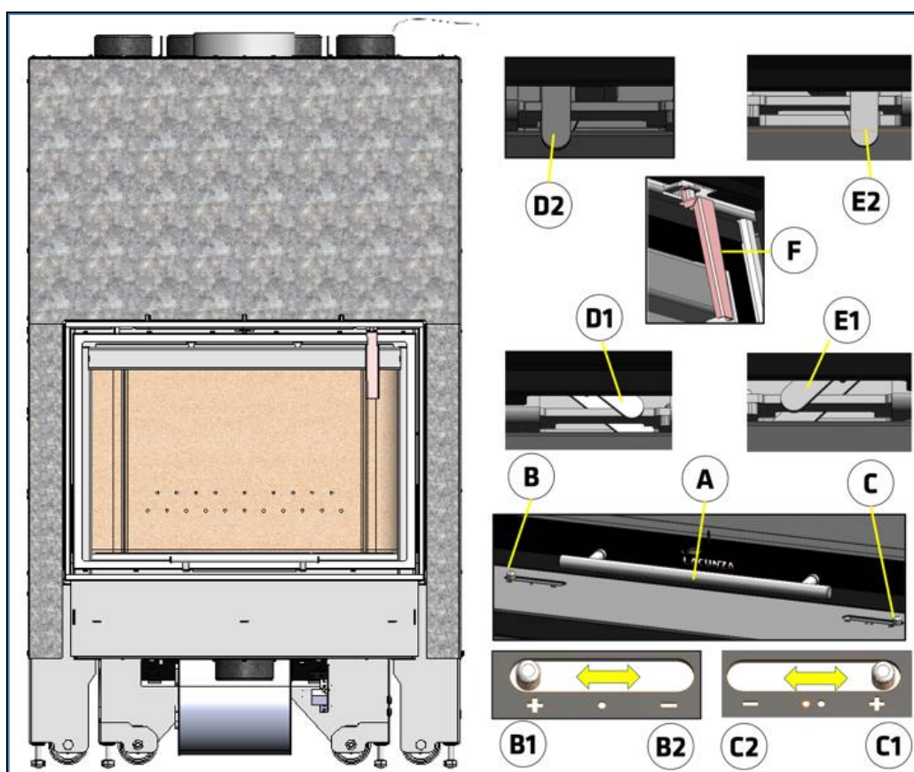
Figura nº26 - Elementos de funcionamento do aparelho
