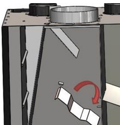
Figura nº33 - Desmontagem do defletor superior Itaca 80
