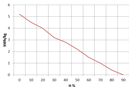
Figura nº25 - Relação entre humidade e poder calorífico da lenha.
