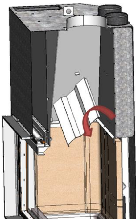
Figura nº35 - Desmontagem do defletor médio Itaca
