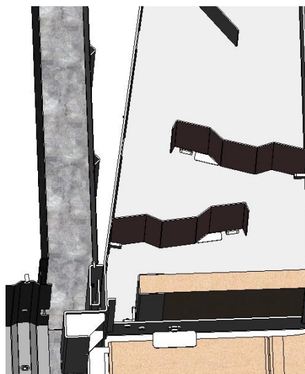
Figura nº29 - Vista de secção Itaca 80 eco com os defletores instalados
