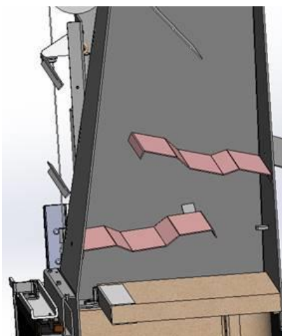
Figura nº27 - Posição atual dos defletores
