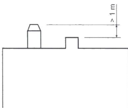
Figura nº22 - Distâncias desde o acabamento até à cumeeira do telhado
