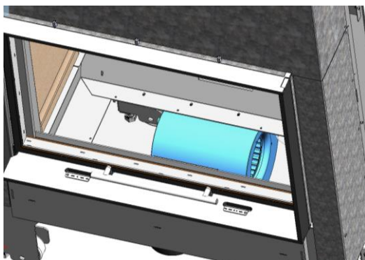
Figura nº47 - Acesso à turbina pelo interior da lareira
