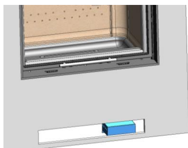
Figura nº19 - Posicionamento do módulo de potência em frente à grade de ventilação frontal
