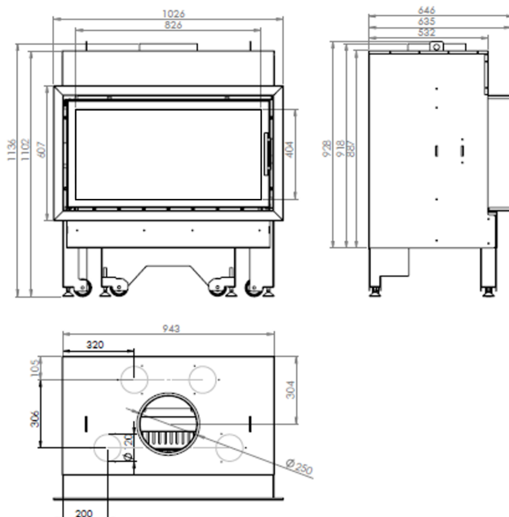
Figura nº2 - Dimensões em mm do aparelho Inca 100
