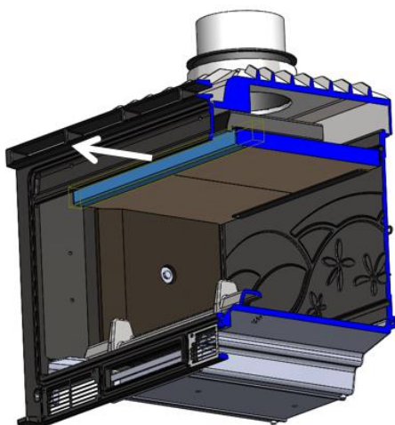
Figura nº12 - Remover o reforço
