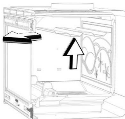
Figura nº11 - Vista de seção do defletor na posição
