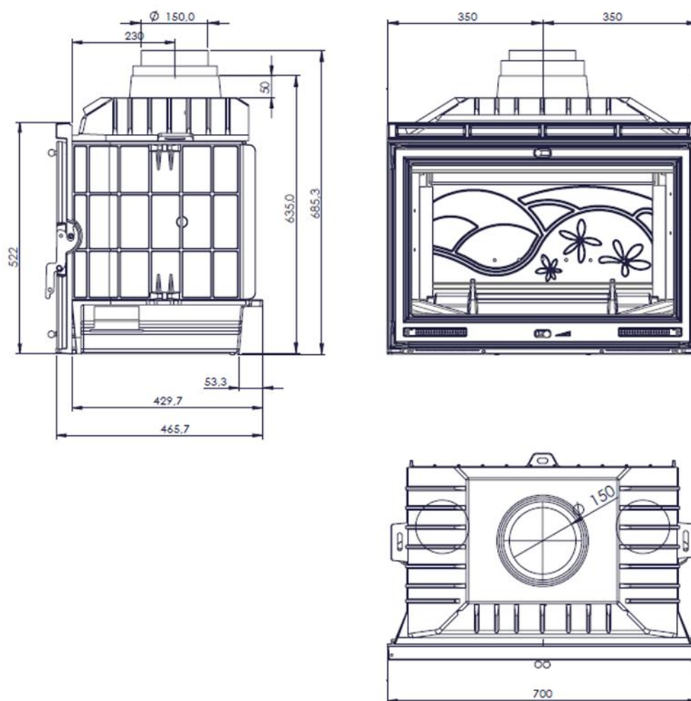
Figura nº2 - Dimensões em mm do aparelho RE-700/NEPAL
