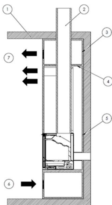
Figura nº4 - Esquema interior do fecho
