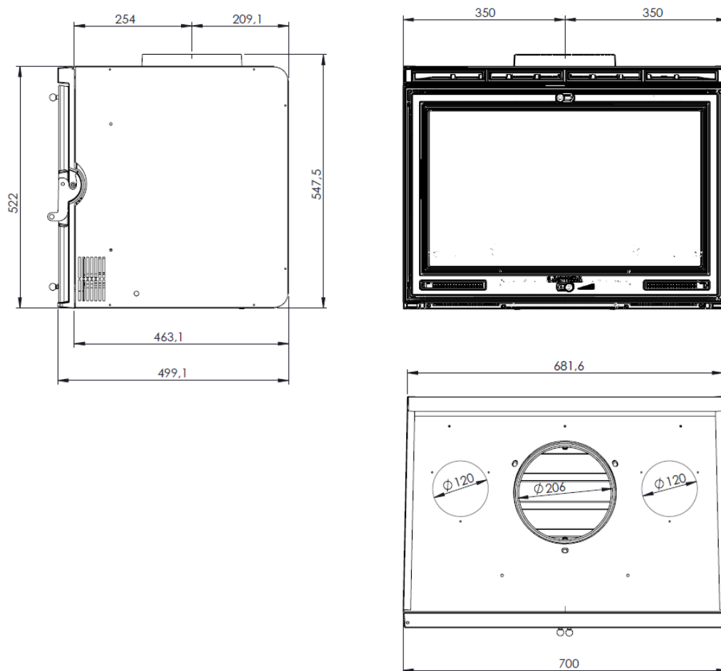
Figura nº1 - Dimensões em mm do aparelho IN-700/INDIA
