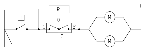
Figura nº15 - Esquema elétrico das ventoinhas
