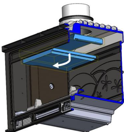
Figura nº13 - Trazer para a frente e inclinar uma metade do deflector de vermiculite para o remover
