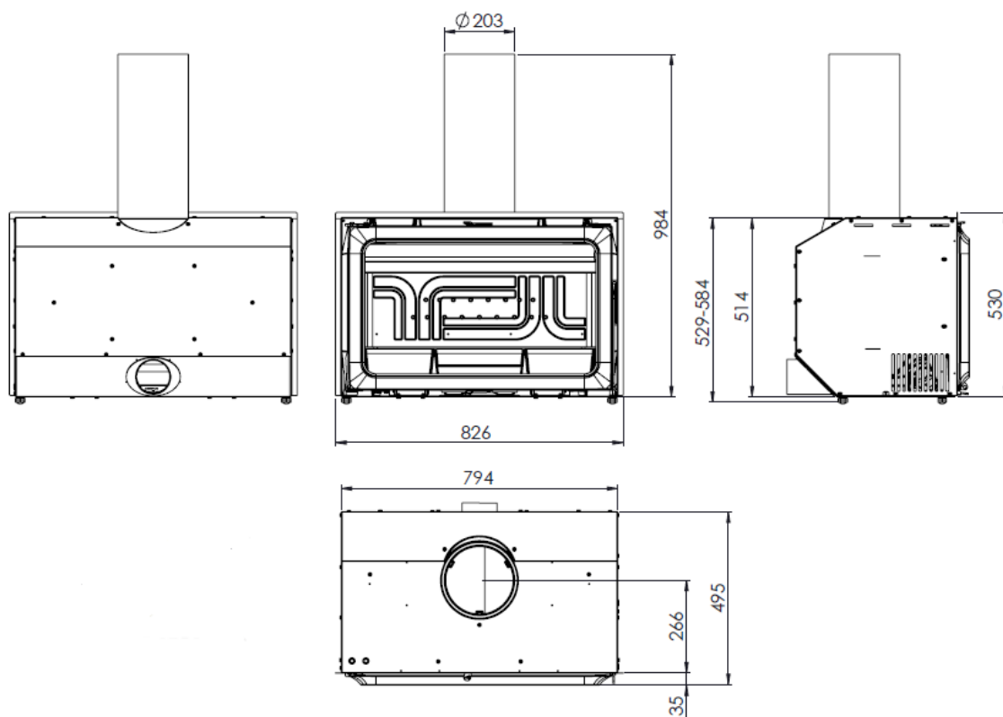
Figura nº1 - Dimensões em mm do aparelho IF-800
