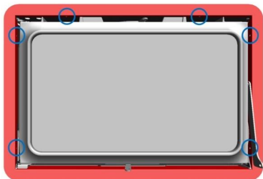
Figura nº10 - Pontos de fixação dos parafusos
