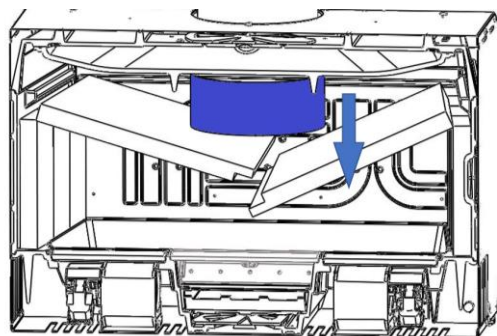
Figura nº27 - Remoção do deflector curvo
