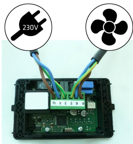
Figura nº14 - Ligações a realizar no potenciômetro
