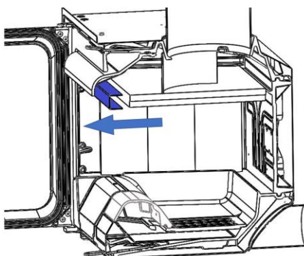
Figura nº25 - Desmontagem do reforço
