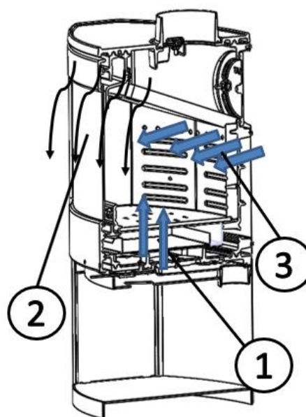
Figura nº19 - Entradas de ar de combustão
