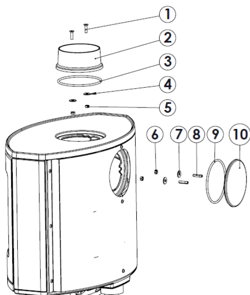
Figura nº9 - Desmontagem de tampa traseira e anel de ligação superior
