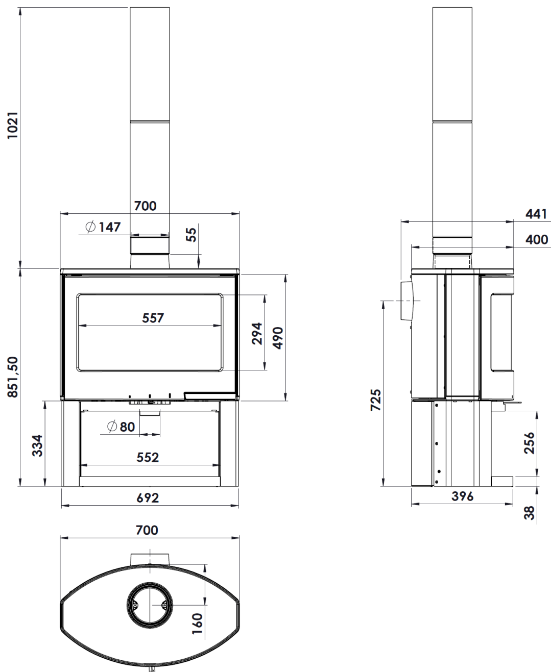
Figura nº1 - Dimensões em mm do aparelho Dublin Star / Bristol Star
