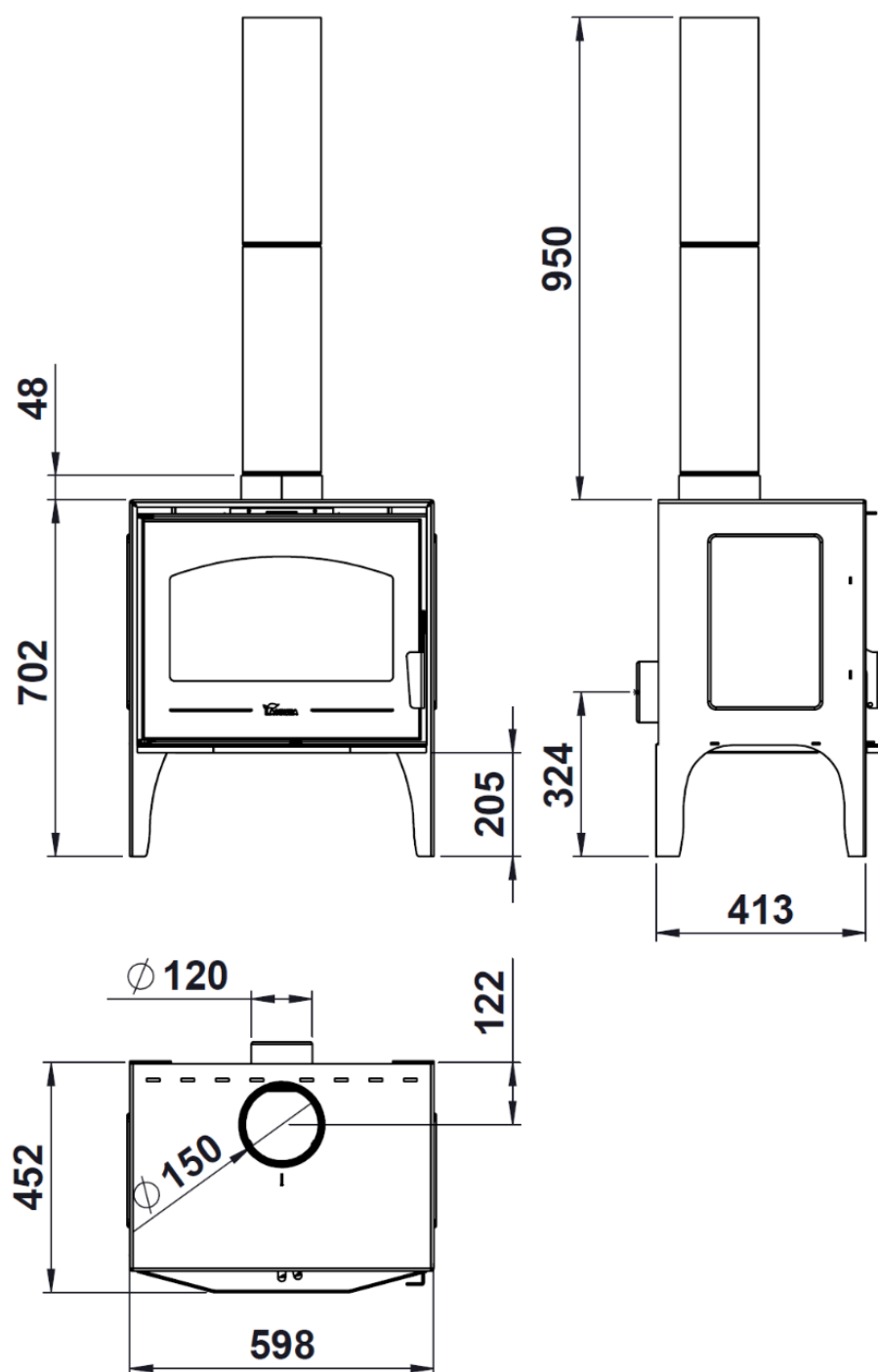
Figura nº1 - Dimensões em mm do aparelho CALPE STAR
