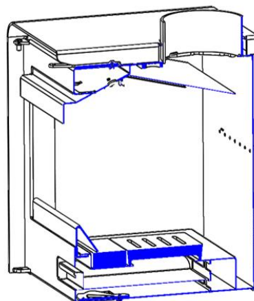
Figura nº13 - Extraía o restante das vermiculites
