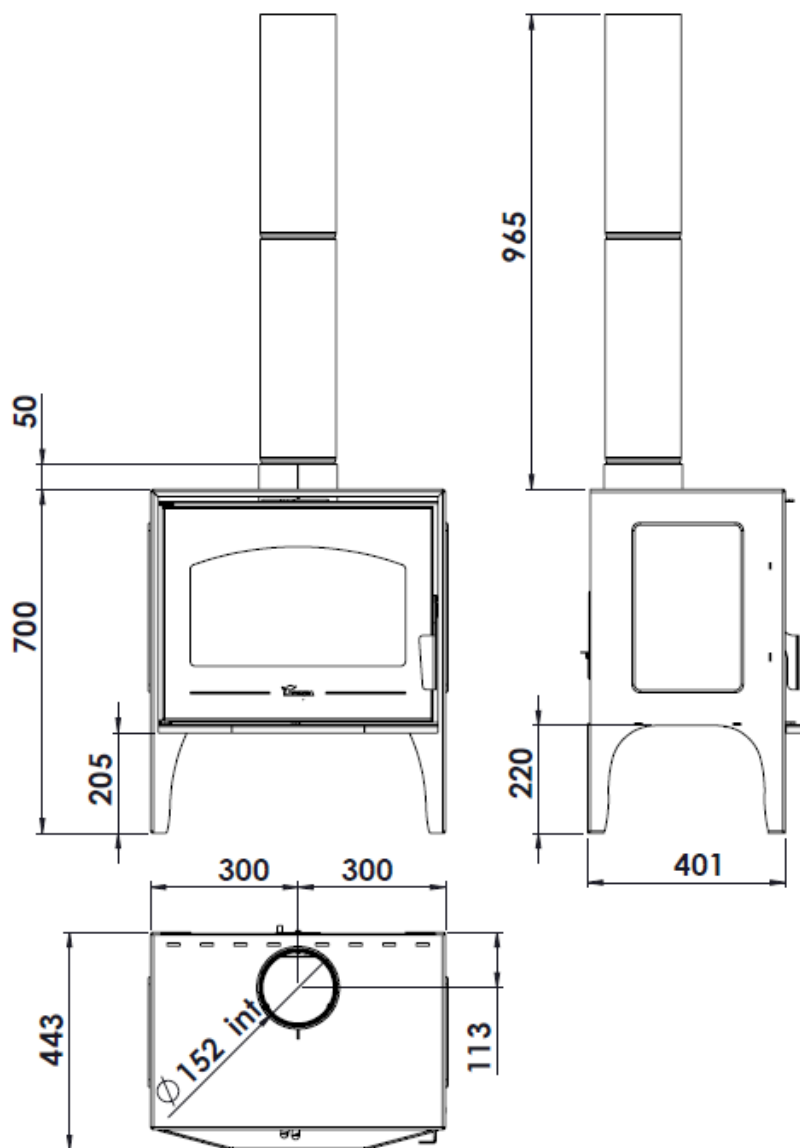
Figura nº1 - Dimensões em mm do aparelho CALPE
