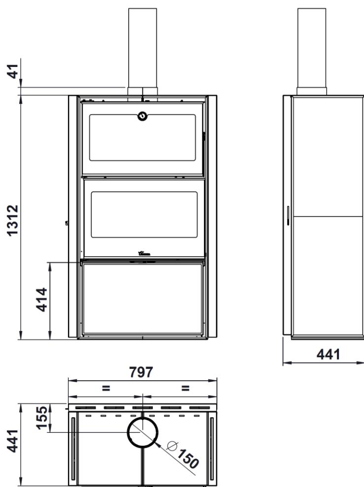
Figura nº1 - Dimensões em mm do aparelho BERGEN
