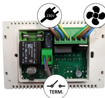
Figura nº10 - Ligações a realizar no potenciômetro
