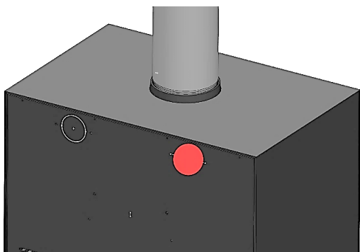
Figura nº13 - Remover a chapa circular
