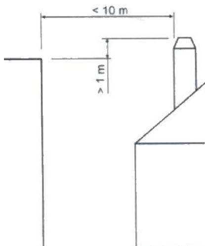
Figura nº21 - Distâncias desde o acabamento até objetos a menos de 10m
