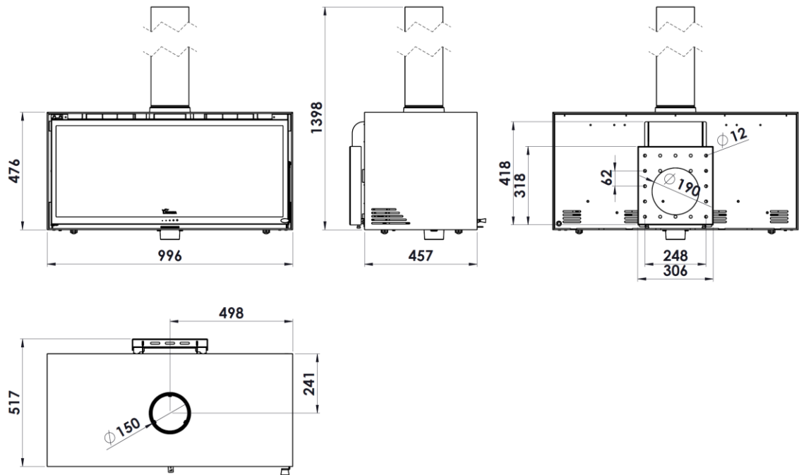
Figura n°6 - Dimensões em mm do aparelho BAIONA 1000 MURAL
