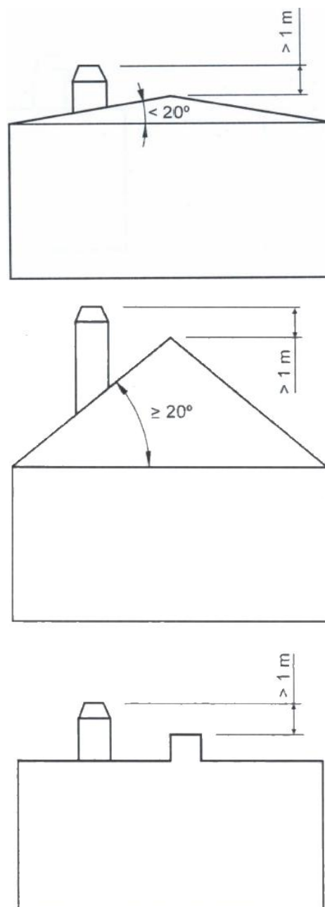
Figura nº20 - Distâncias desde o acabamento até à cumeeira do telhado
