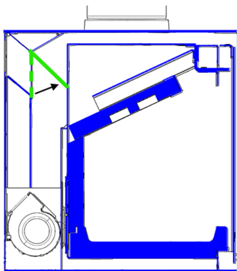
Figura nº18 - Empurre a chapa interior até ao batente
