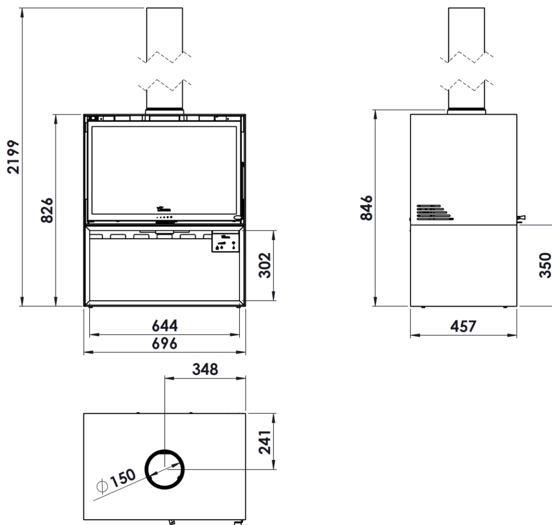
Figura nº1 - Dimensões em mm do aparelho BAIONA 700
