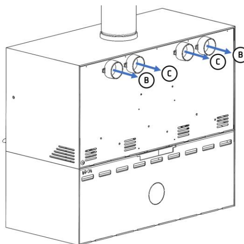
Figura nº9 - Baiona 1000
