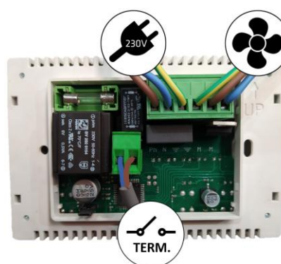
Figura nº7 - Ligações a realizar no potenciômetro
