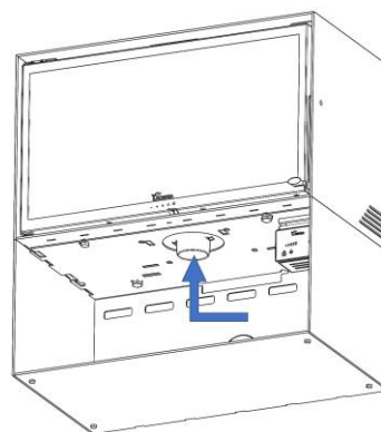
Figura nº5 - Condução de ar para câmara de combustão
