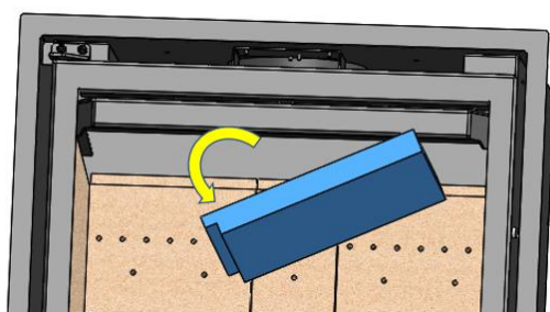
Figura nº23 - Desmontagem defletor
