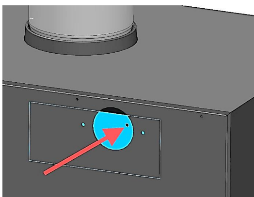
Figura nº12 - Mude a posição da chapa interior empurrando-a para dentro
