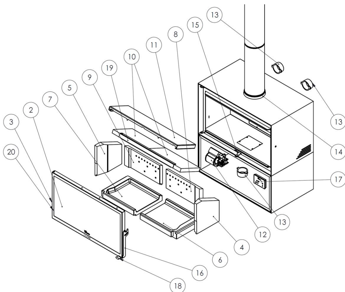
Figura nº25 - Baiona 700-800
