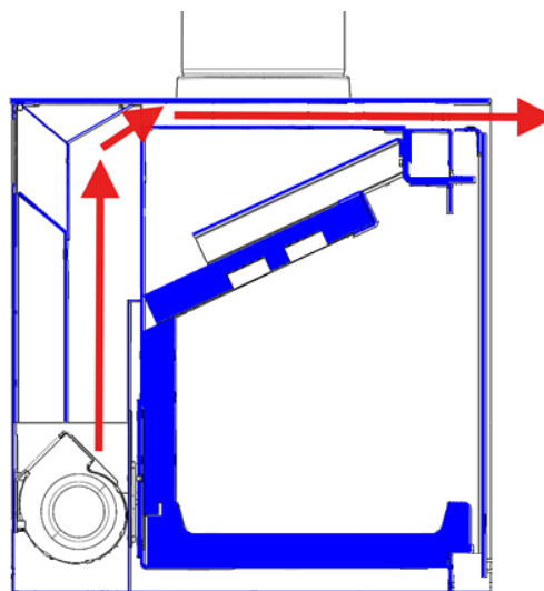
Figura nº14 - Percurso do ar quente sem canalizações
