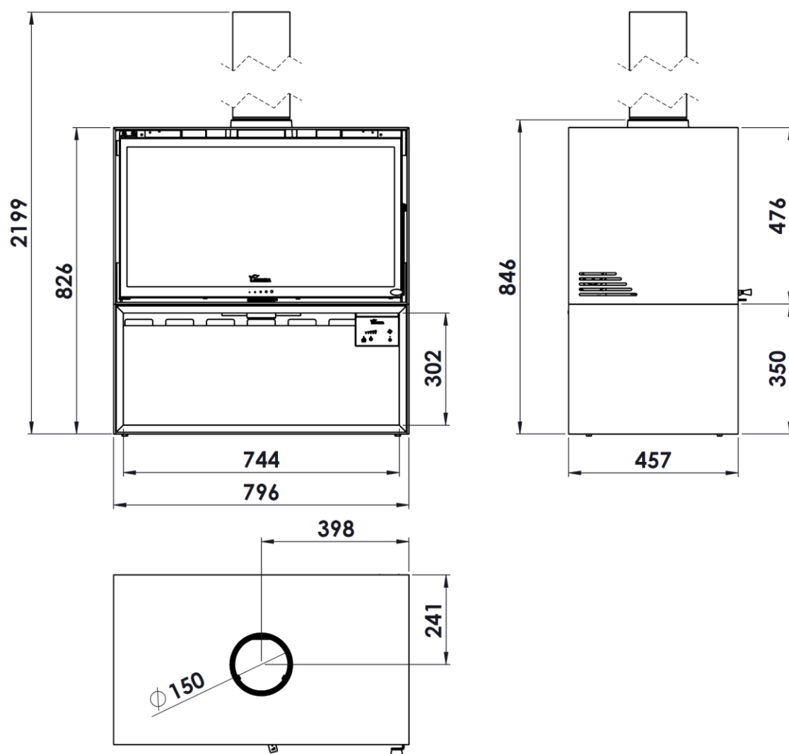
Figura nº2 - Dimensões em mm do aparelho BAIONA 800
