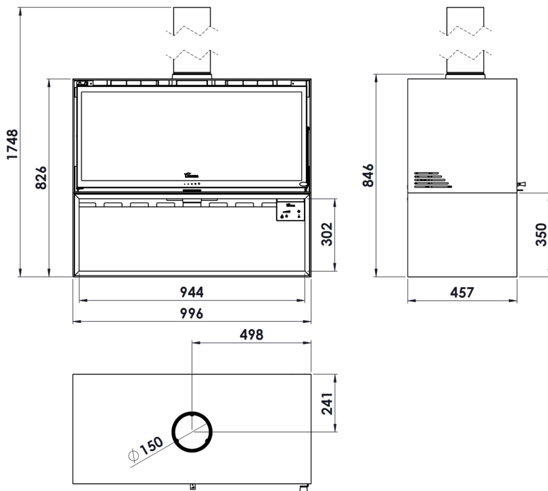
Figura nº3 - Dimensões em mm do aparelho BAIONA 1000
