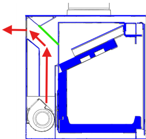
Figura nº16 - Trajetória do ar quente com canalização
