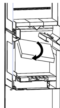
Figura nº14 - Extração dos defletores de vermiculita
