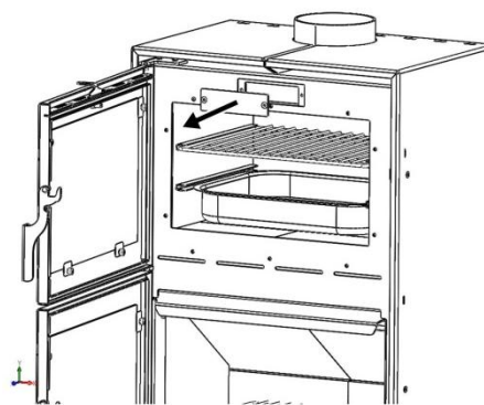
Figura nº18 - Retirada das tampas de acesso
