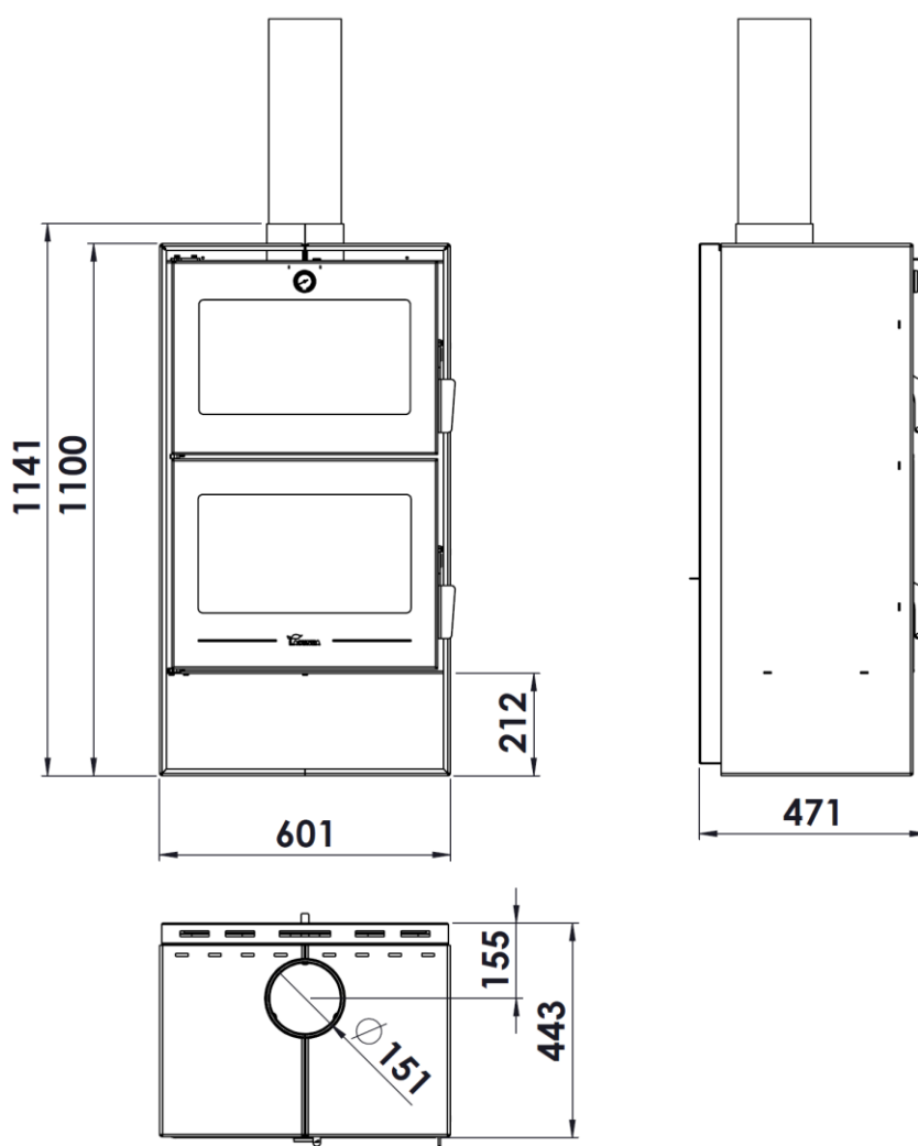
Figura nº1 - Dimensões em mm do aparelho ALTEA
