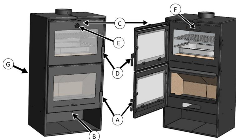
Figura nº7 - Elementos de funcionamento do aparelho
