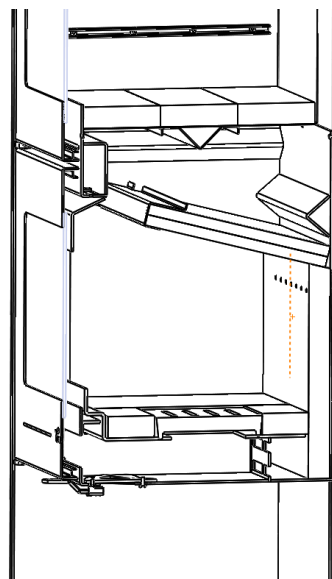
Figura nº17 - Reforço de aço inoxidável na posição aberta
