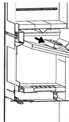
Figura nº13 - Reforço sobre os defletores de vermiculita
