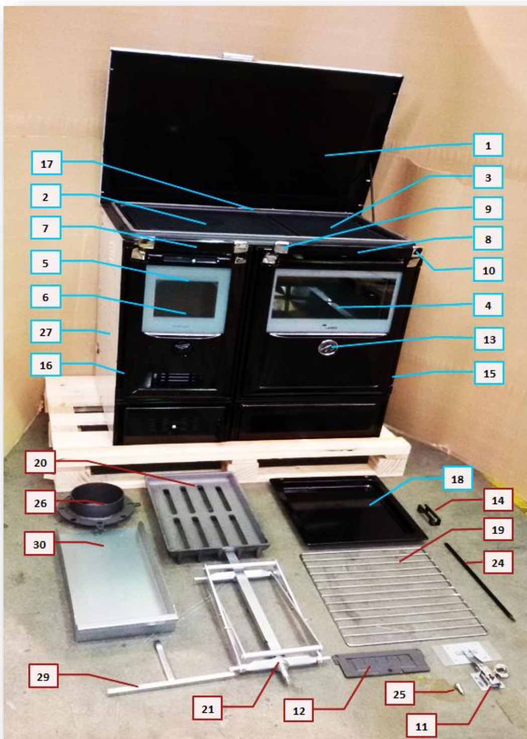
Figura nº26 - Despiece básico del aparato
