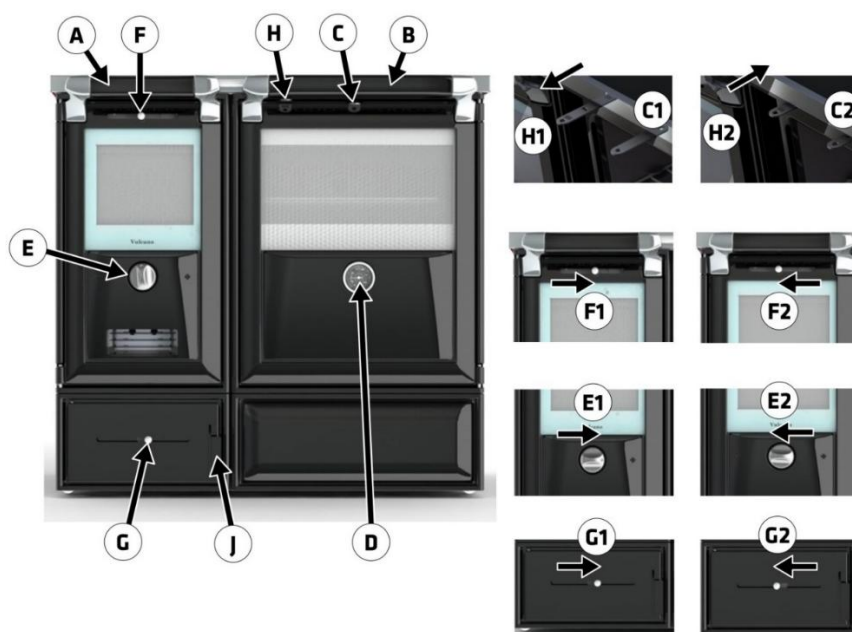
Figura nº14 - Elementos de funcionamiento del aparato
