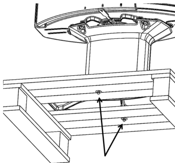
Figura nº6 - Detalle de los tornillos que amarran la estufa a la base de madera
