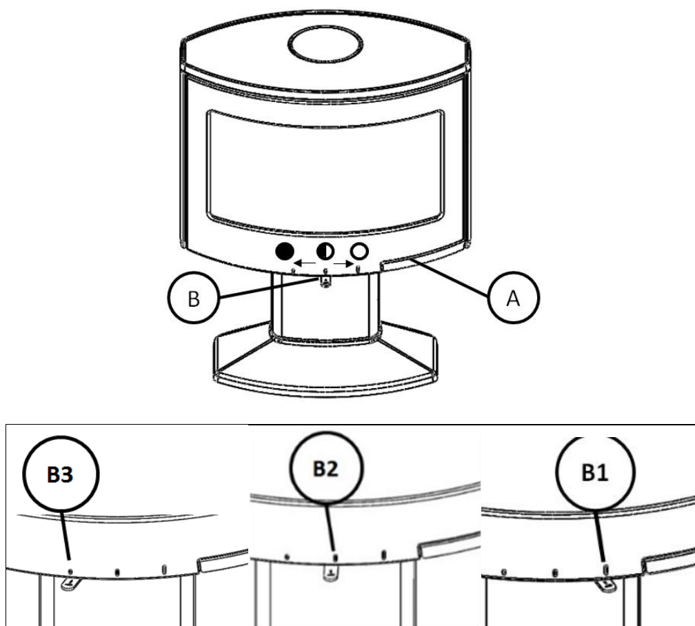
Figura n°15 - Elementos de funcionamiento del aparato
