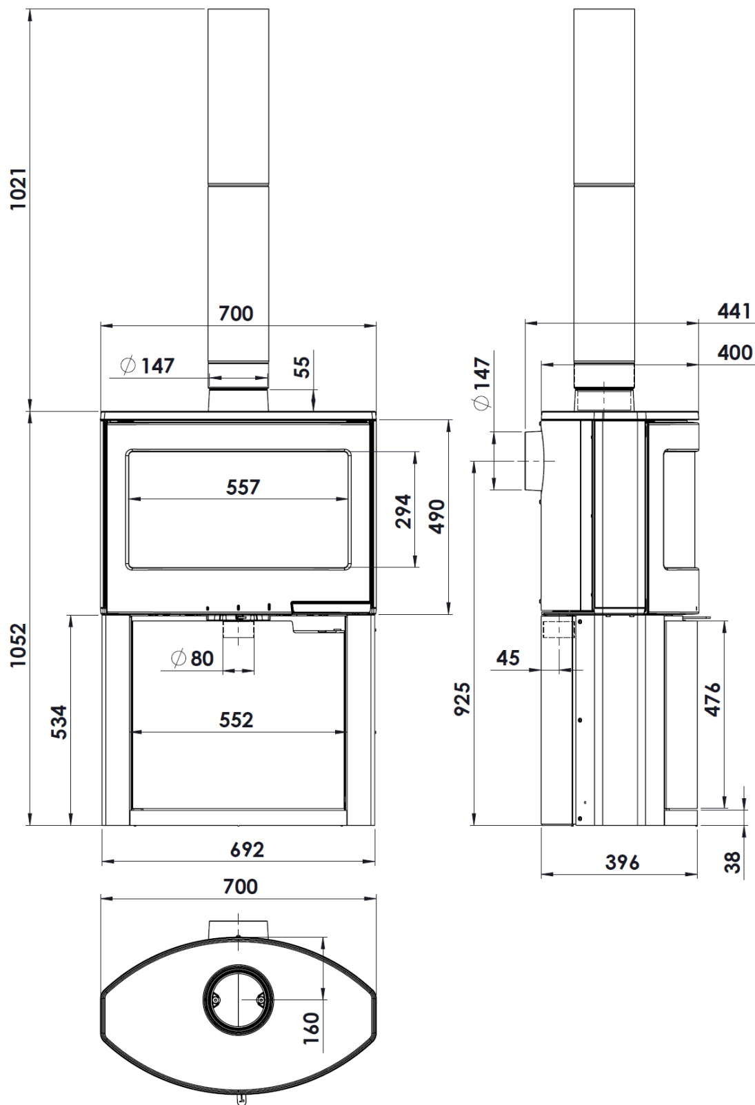
Abbildung Nr.3- Abmessungen des Geräts in mm Bera Star
