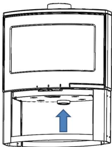
Abbildung Nr.10- Luftkanal für die Brennkammer, Tarbes Star-Bristol Star.
