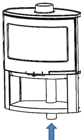
OPTION 2: Außenluftführung im BRISTOL STAR-Ofen
