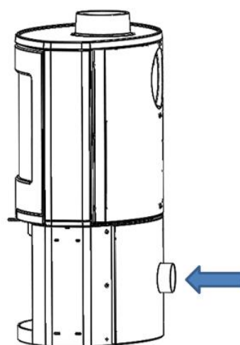
OPTION 1: Außenluftführung im BRISTOL STAR-Ofen
