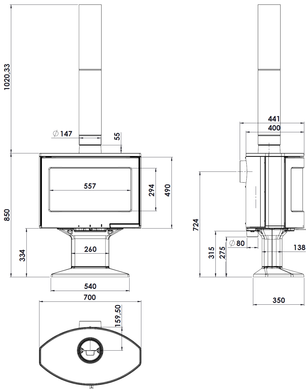
Abbildung Nr.1 - Abmessungen des Geräts in mm Tarbes Star
