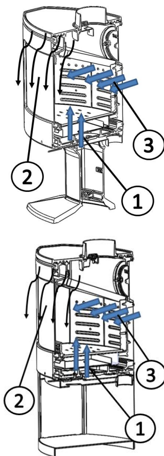
Abbildung Nr.16- Verbrennungslufteinlässe
