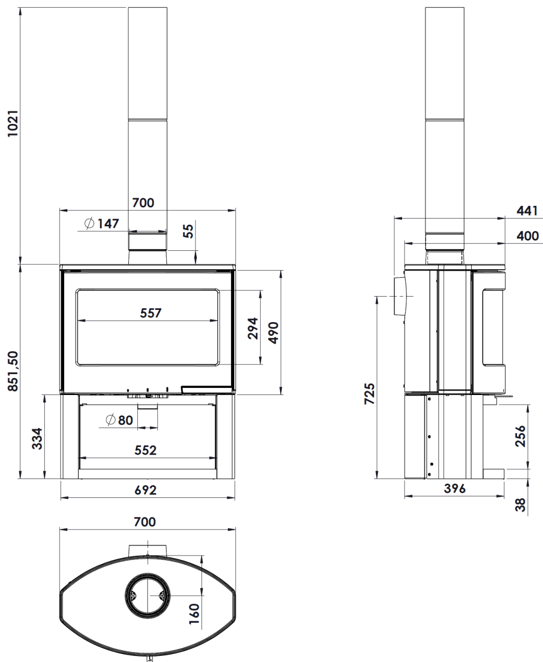
Abbildung Nr.2 - Abmessungen des Geräts in mm Bristol Star
