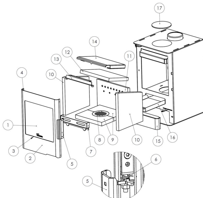
Figura nº23 - Despiece NOMAD
