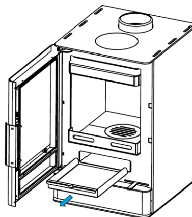
Figura nº11 - Extracción del cenicero
