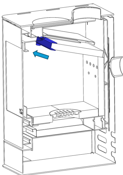
Figura n°12 - Extraer refuerzo
