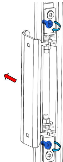
Figura n°21 - PASO 2: Apretar los tornillos que regulan la profundidad hasta donde nos interese
