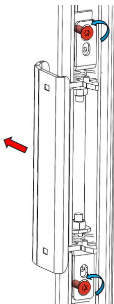
Figura n°20 - PASO 1: Aflojar tornillos
