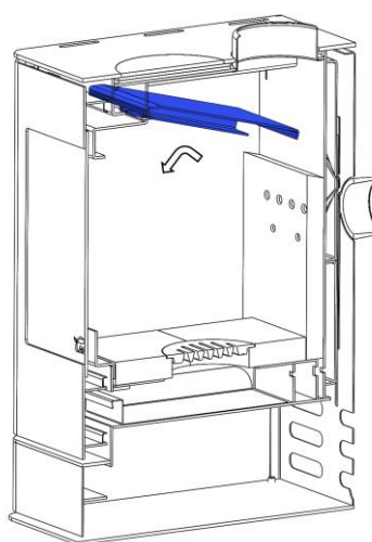
Figura n°15 - Desmontar deflector chapa
