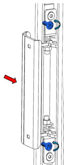
Figura n°18 - PASO 2: Aflojar los tornillos que regulan la profundidad hasta donde nos interese
