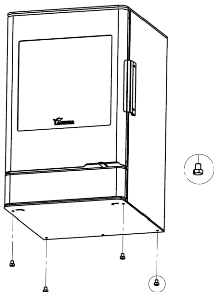
Figura n°16 - Instalación patas nivelación
