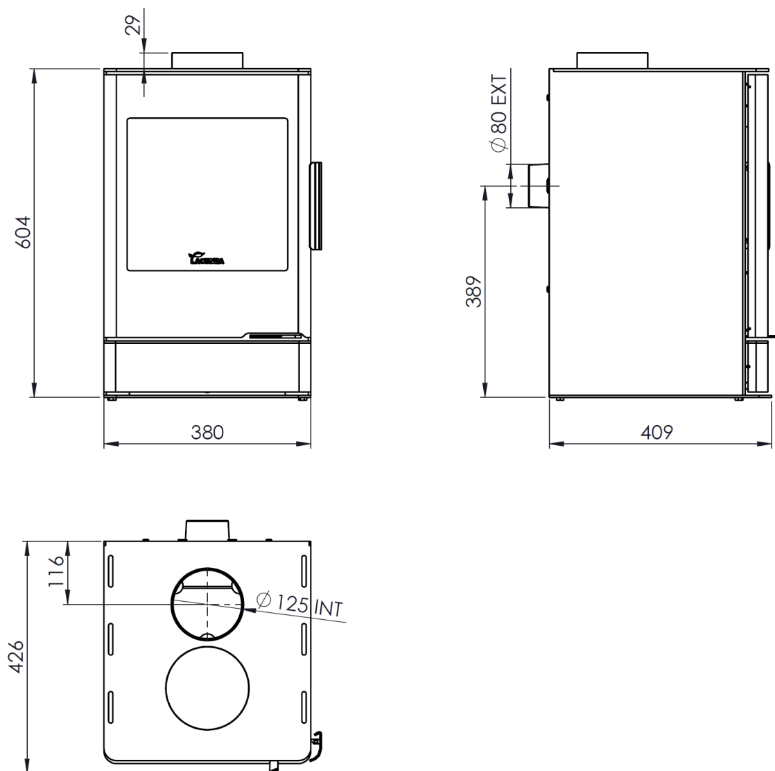
Figura n°1 - Dimensiones en mm de NOMAD
