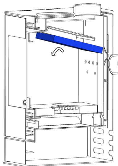
Figura n°14 - Desmontar deflector vermiculita
