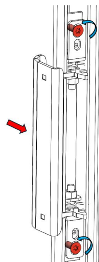
Figura n°17 - PASO 1: Aflojar tornillos
