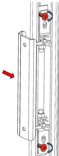
Figura n°19 - PASO 3: Apretar tornillos para volver a fijar el sistema
