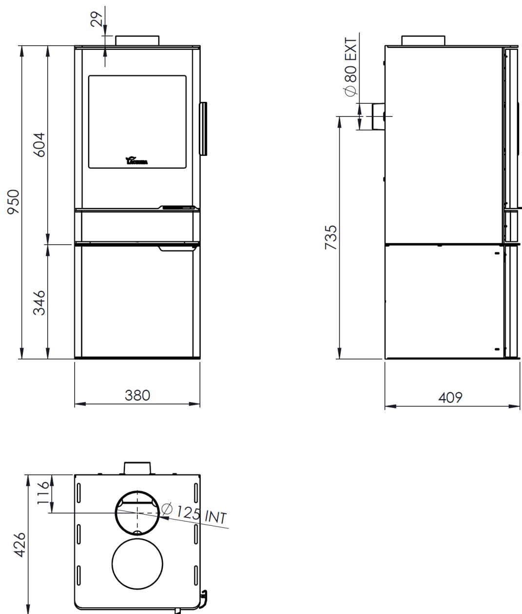
Figura n°2 - Dimensiones en mm de NOMAD con Accesorio
