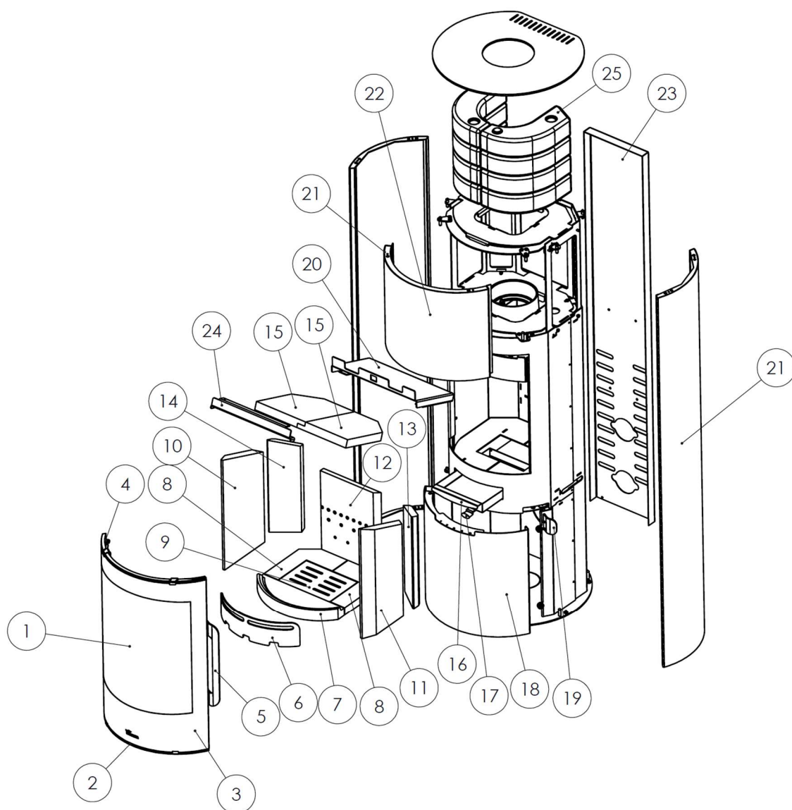
Figura nº4 - Despiece MAYA ACU Visión
