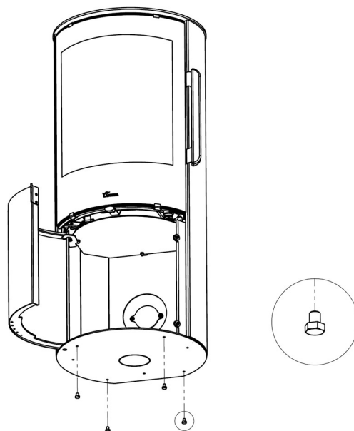
Figura n°19 - Instalación patas nivelación
