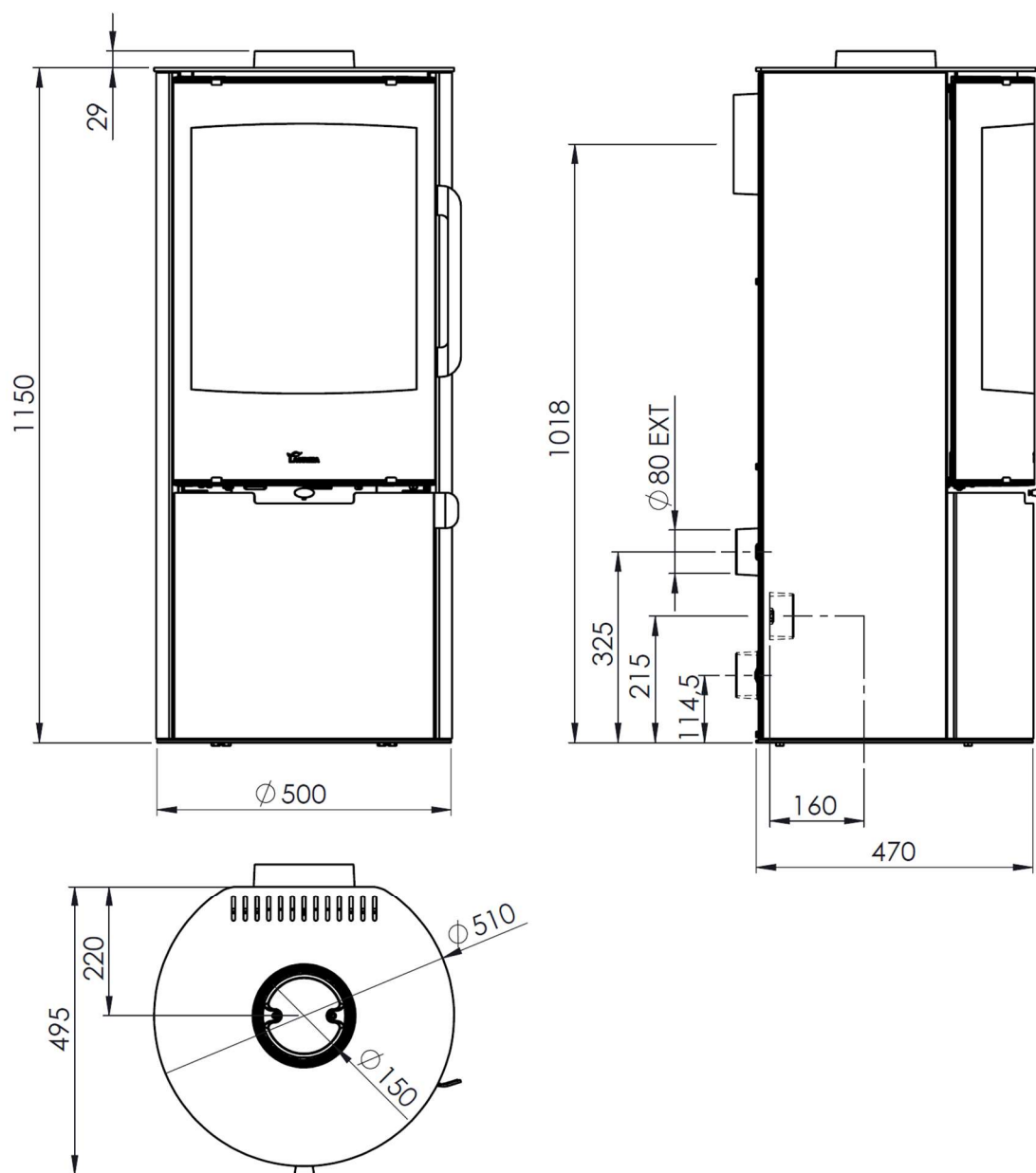
Figura nº1 - Dimensiones en mm de MAYA y MAYA Visión
