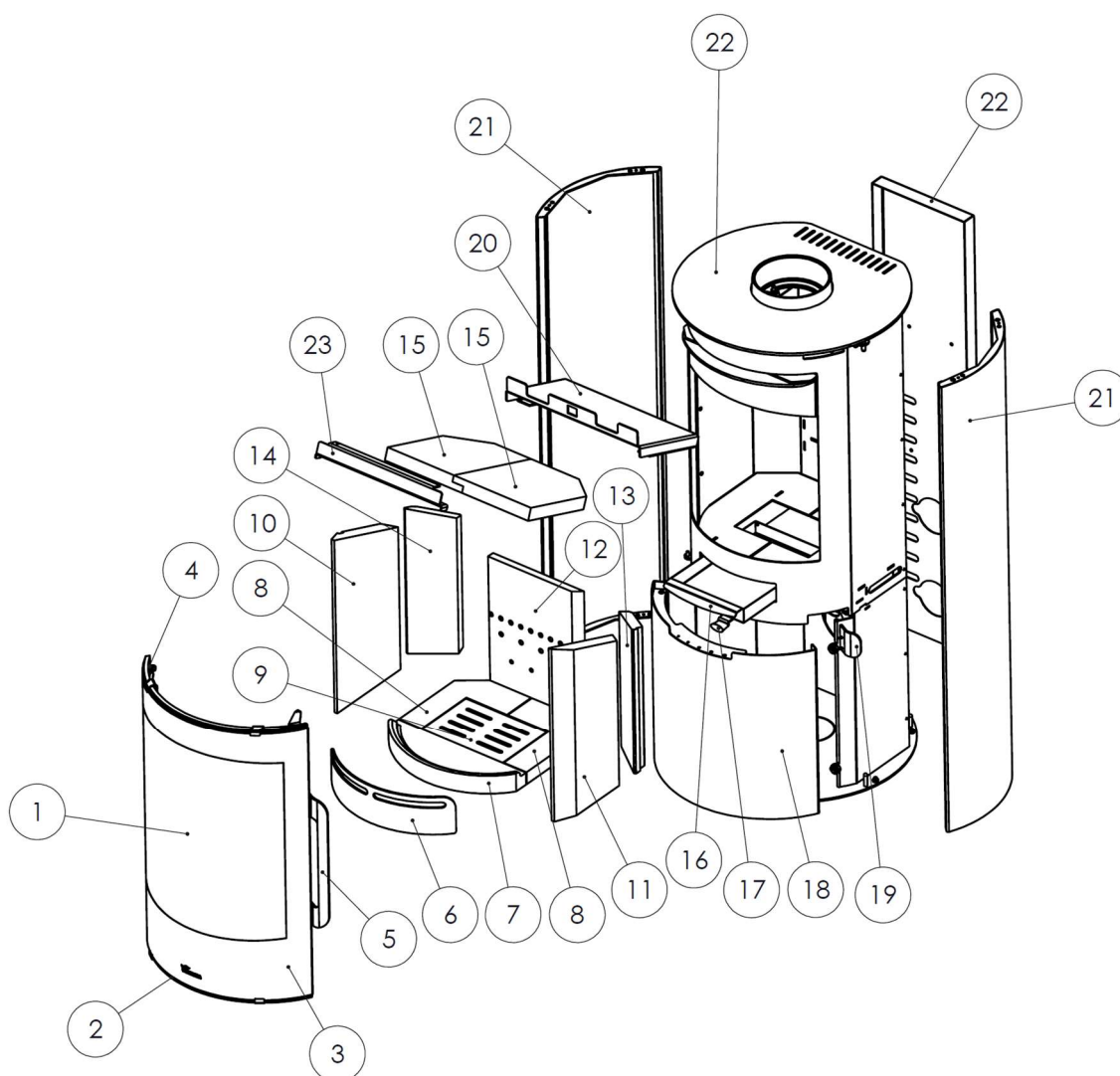
Figura n°2 - Despiece MAYA Visión
