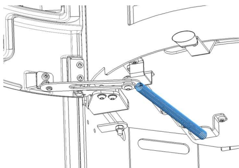
Figura n°20 - Paso 1. Desmontar muelle
