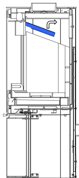
Figura n°18 - Desmontar deflector acero
