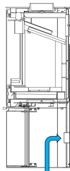
Figura nº9 - OPCIÓN 3 Conducción de aire para cámara de combustión
