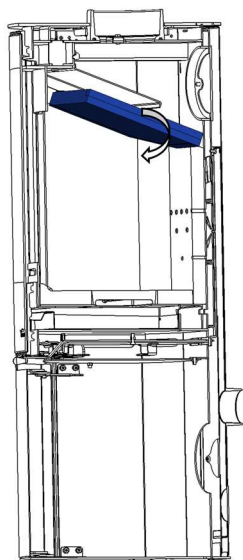
Figura n°17 - Retirar vermiculita
