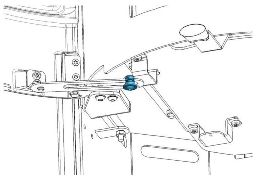
Figura n°21 - Paso 2. Desmontar eje
