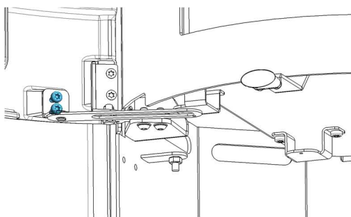
Figura n°22 - Paso 3. Desmontar tornillos soporte puerta
