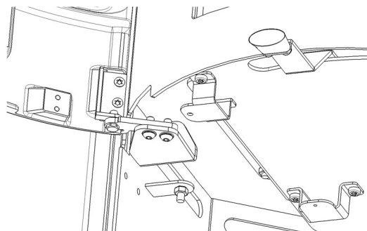
Figura n°23 - Paso 4. Quitar mecanismo
