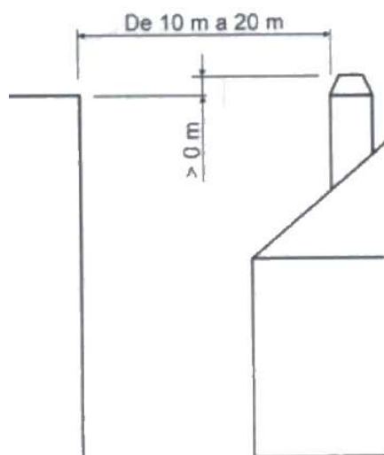
Figura n°12 - Distancias desde el remate hasta objetos entre 10 y 20m
