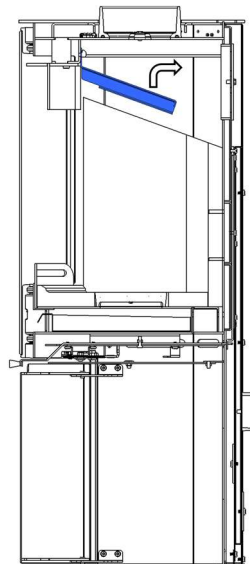
Figura nº18 - Desmontar deflector acero
