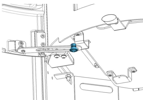
Figura nº20 - Paso 1. Desmontar muelle
