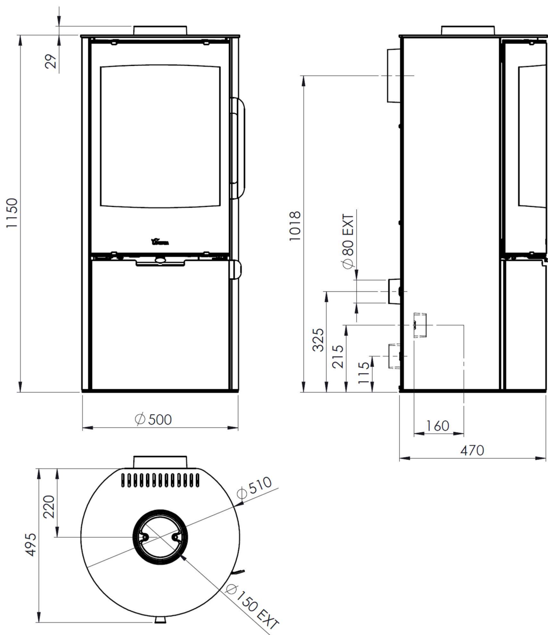
Figura nº1 - Dimensiones en mm de MAYA y MAYA Visión
