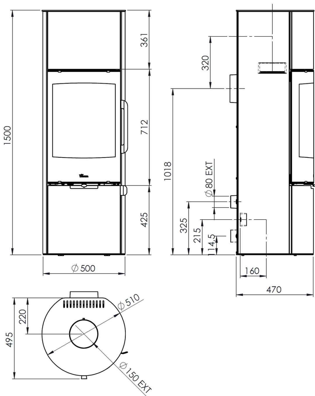
Figura nº2 - Dimensiones en mm de MAYA ACU y MAYA ACU Visión
