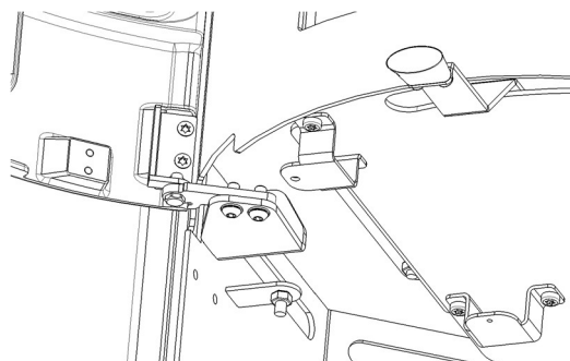
Figura nº23 - Paso 4. Quitar mecanismo
