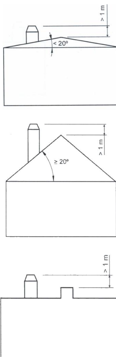
Figura nº17 - Distancias desde el remate hasta la cumbrera del tejado
