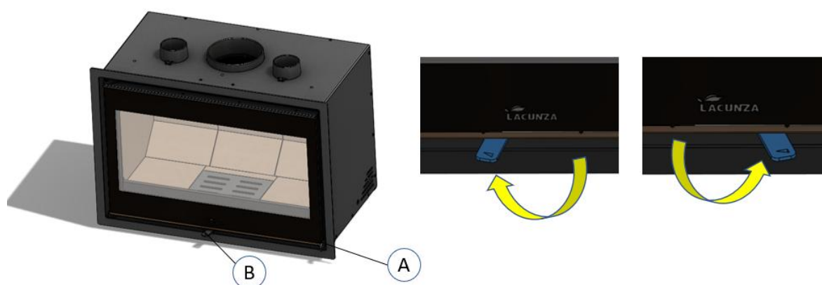
Figura n°21 - Elementos de funcionamiento del aparato
