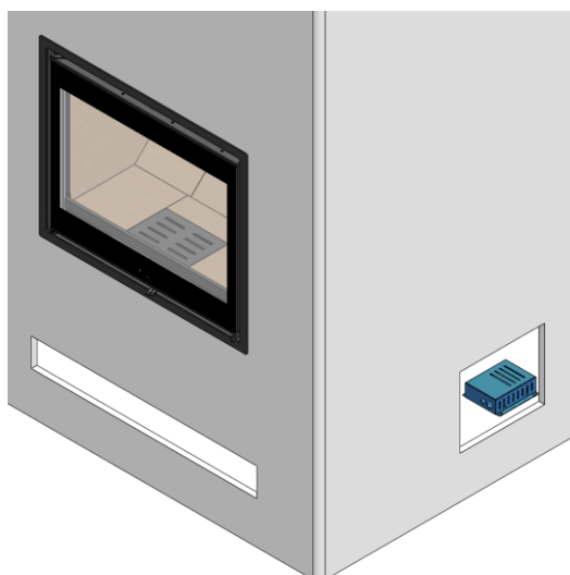
Figura n°16 - Posicionamiento de la carcasa del regulador frente a la rejilla de ventilación lateral
