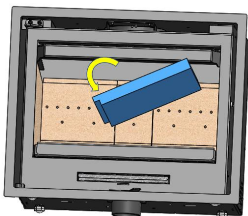
Figura n°23 - Desmontaje de los deflectores inferiores de vermiculita.
