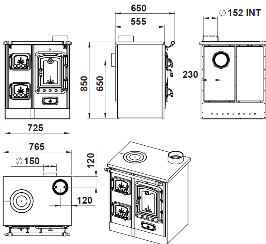
Figura nº1 - Dimensiones en mm del aparato Lis 5T
