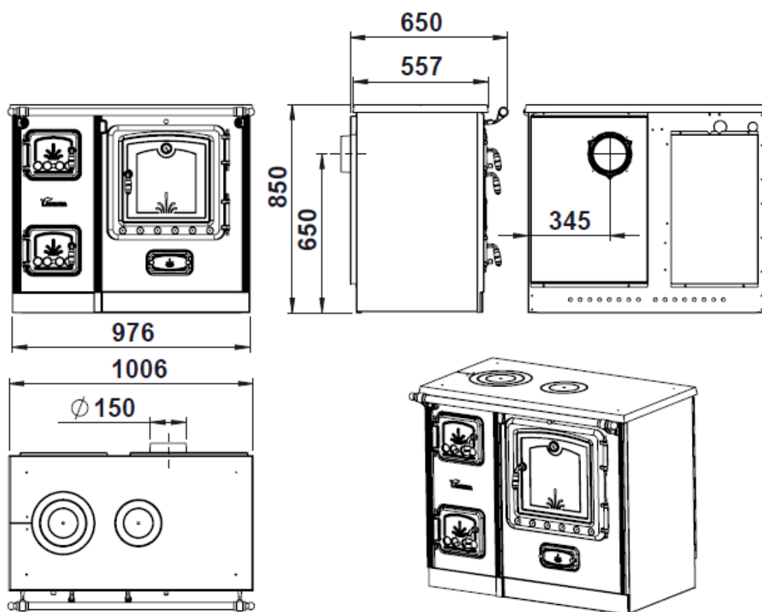
Figura nº3 - Dimensiones en mm del aparato Lis 8T
