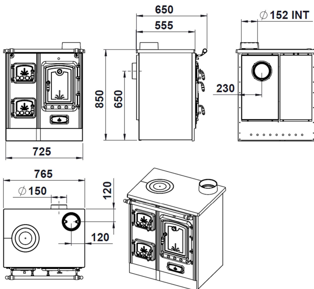
Figura n o 1 - Dimensiones en mm del aparato Lis 5T
