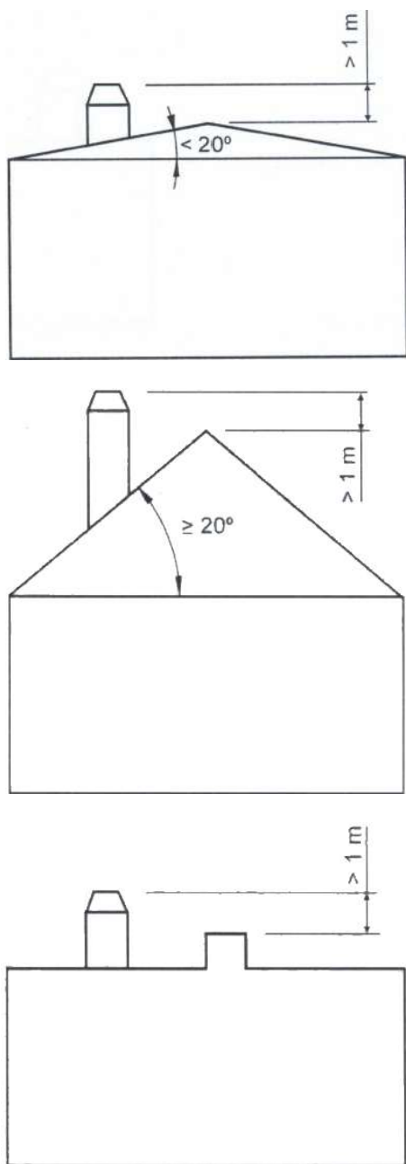
Figura n°9 - Distancias desde el remate hasta la cumbrera del tejado
