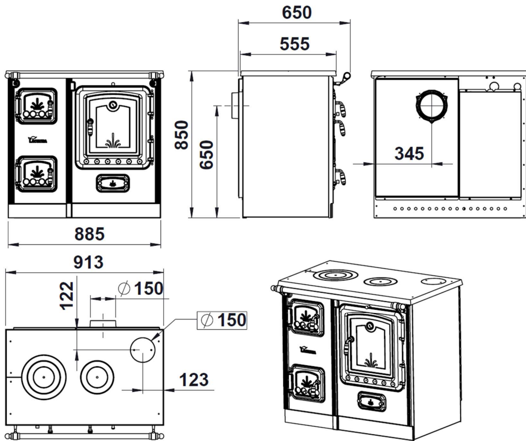
Figura n°2 - Dimensiones en mm del aparato Lis 7T
