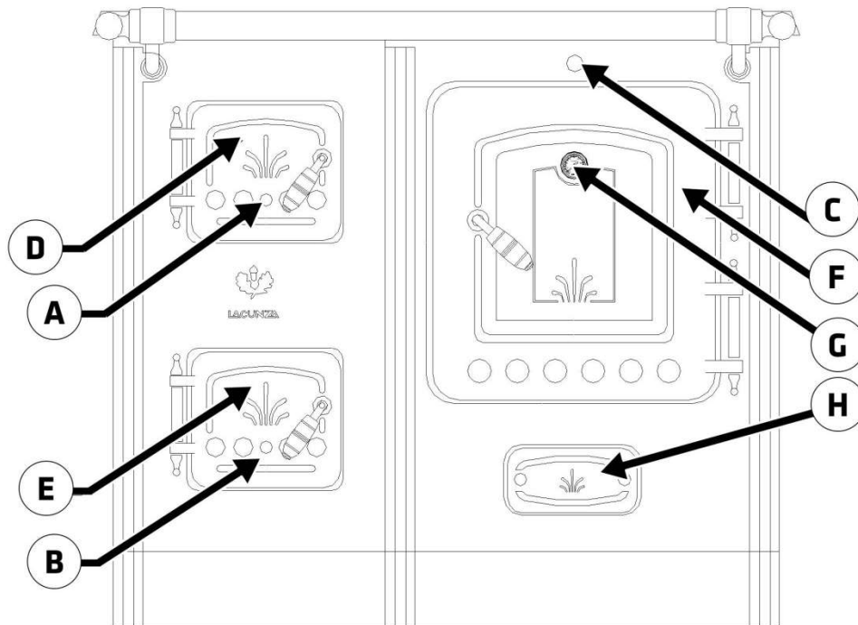
Figura n°13 - Elementos de funcionamiento del aparato
