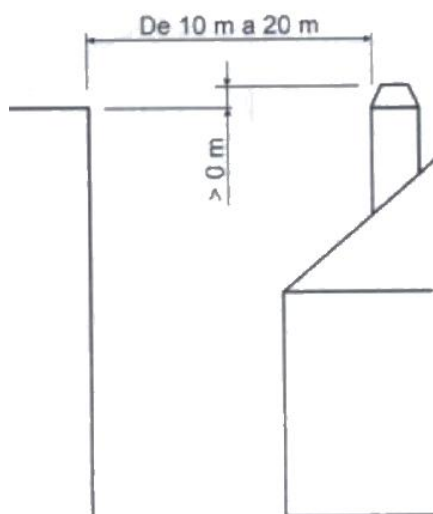
Figura nº27 - Distancias desde el remate hasta objetos entre 10 y 20m
