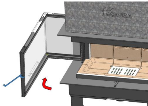
Figura n°43 - Puerta abierta horizontalmente
