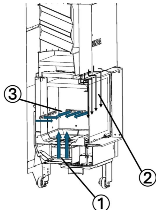
Figura nº32 - Entradas de aire de combustión
