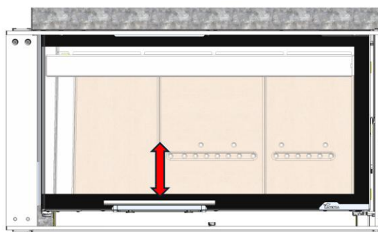
Figura n°38 - Apertura guillotina
