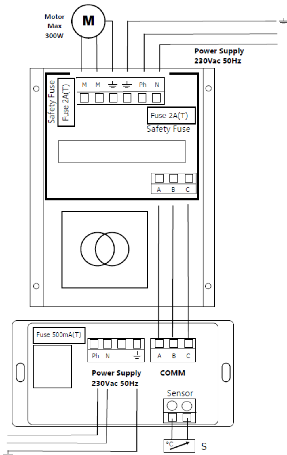
Figura nº20 - Conexiones a realizar en controlador y el módulo de potencia de la Iزارو C/V
