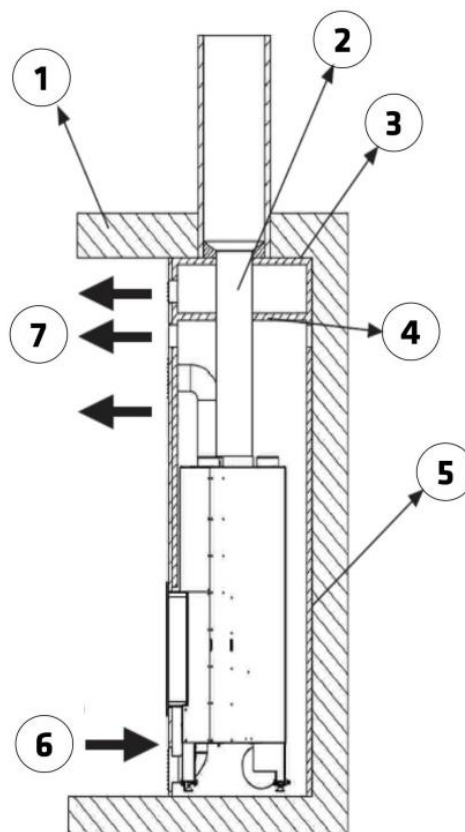
Figura nº9 - Esquema interior del cerramiento
