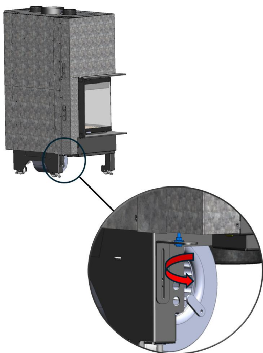
Figura nº7 - Acceso para soltar los tornillos de amarre de los contrapesos IZARO CLI
