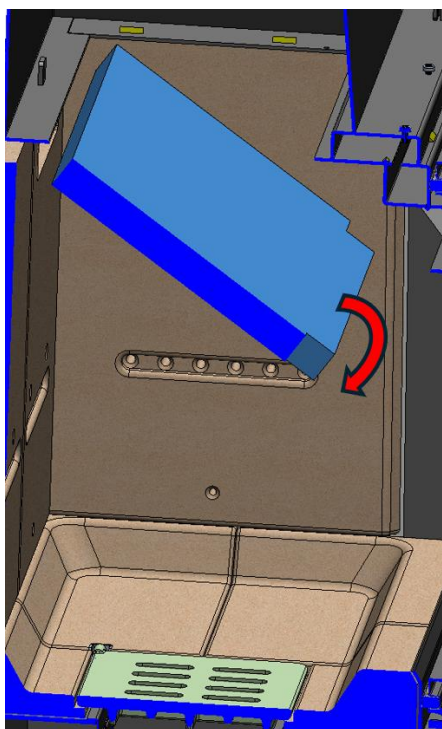
Figura n°37 - Desmontaje del deflector superior Izaro 100 CLI
