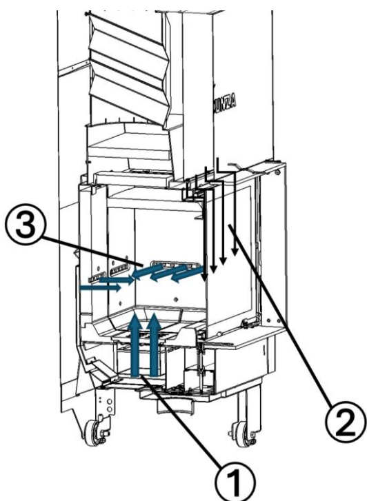
Figura n°32 - Entradas de aire de combustión
