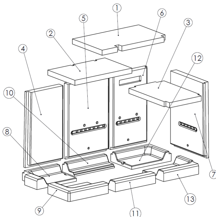
Figura n°50 - Despiece hogar vermi IZARO 100 CLI
