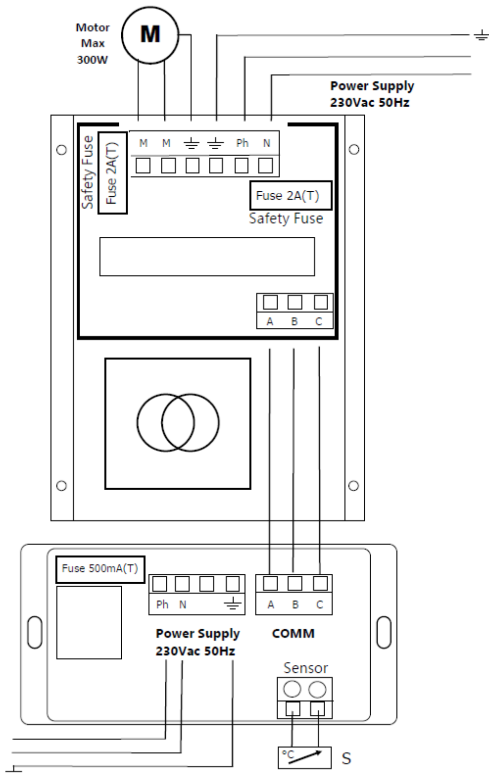
Figura nº20 - Conexiones a realizar en controlador y el módulo de potencia de la Izaro C/V
