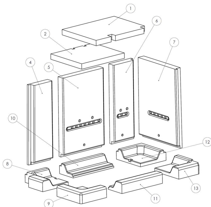
Figura n°49 - Despiece hogar vermi IZARO 80 CLI
