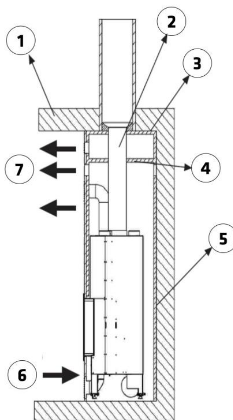
Figura n°9 - Esquema interior del cerramiento
