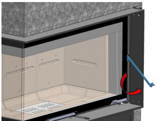
Figura n°42 - Abrir la manilla de la puerta hacia fuera.
