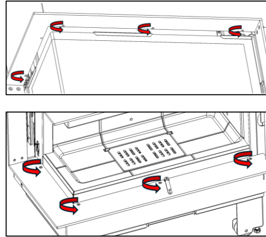
Figura n°17 - Destornillar los 8 tornillos, 4 superiores y 4 inferiores que amarran el marco exterior
