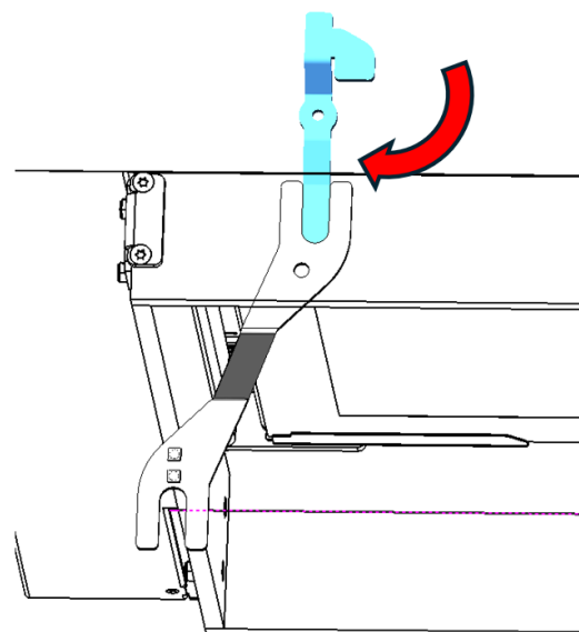
Figura n°41 - Girar la palanca superior-izq en el sentido de agujas reloj 90°
