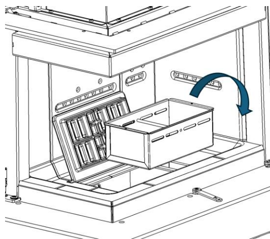
Figura n°33 - Retirada del cajetín cenicero
