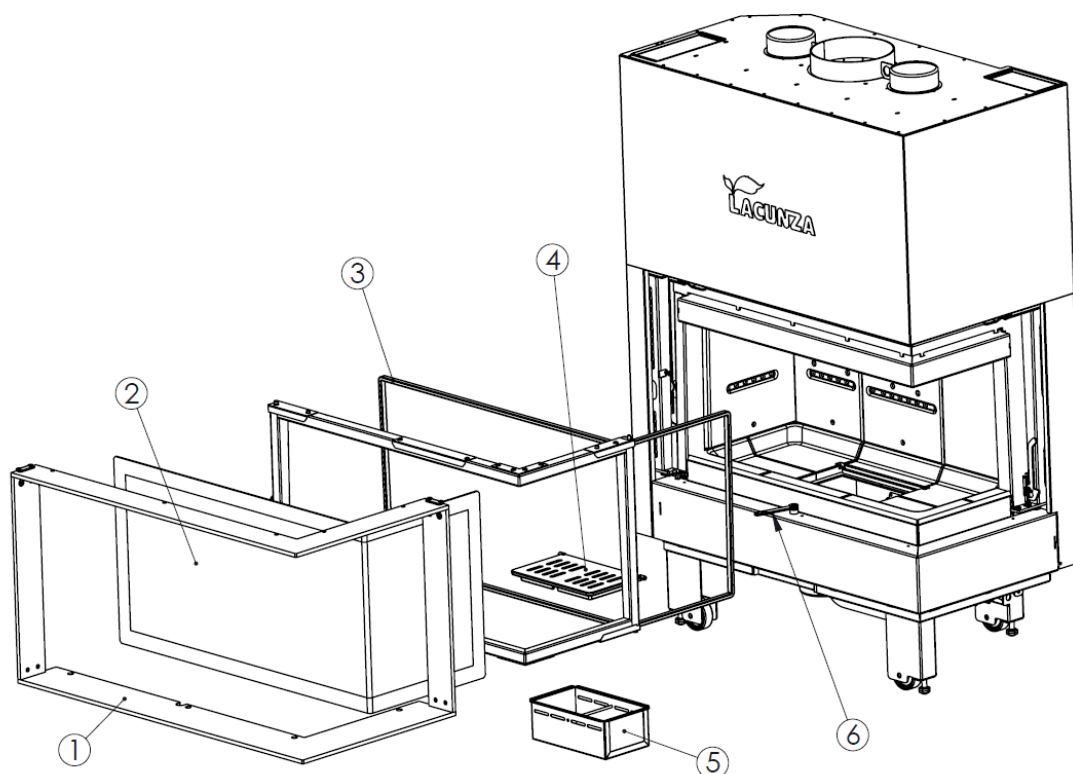
Figura n°51 - Despiece Izaro 80-100 CLD
