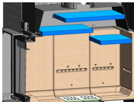
Figura nº34 - Vista de sección Iزارo 100 CLI con los 3 deflectores colocados
