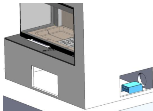
Figura n°23 - Posicionamiento del módulo de potencia frente a la rejilla de ventilación lateral
