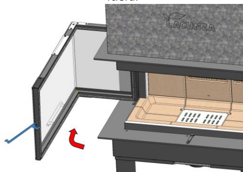
Figura n°43 - Puerta abierta horizontalmente
