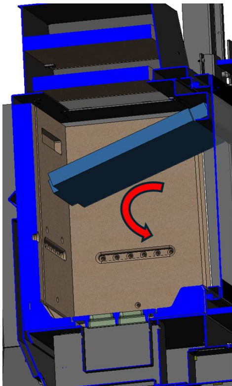
Figura n°35 - Desmontaje del deflector inferior Izaro 100 CLI
