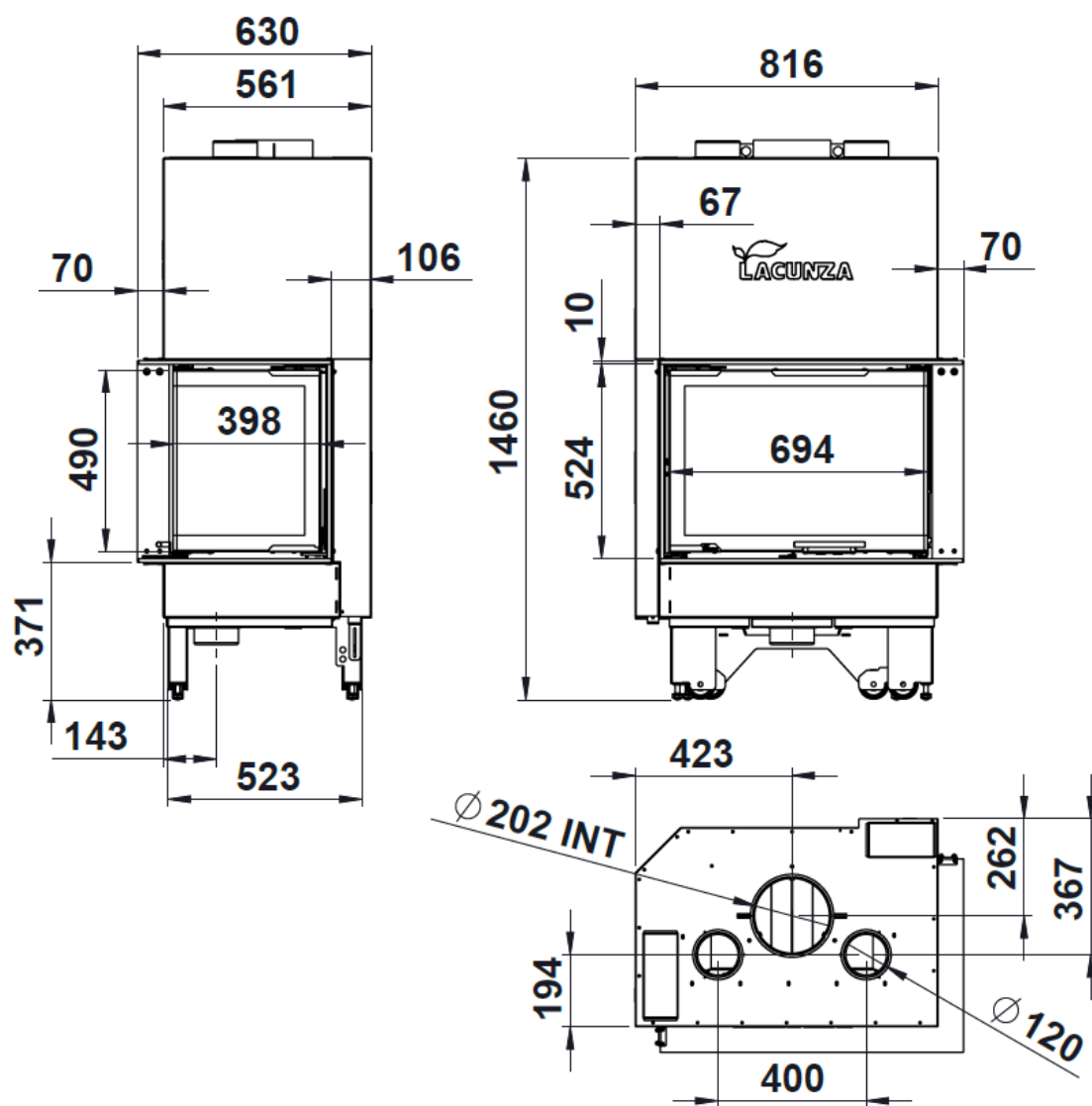
Figura nº3 - Dimensiones en mm del aparato IZARO 80 CLD
