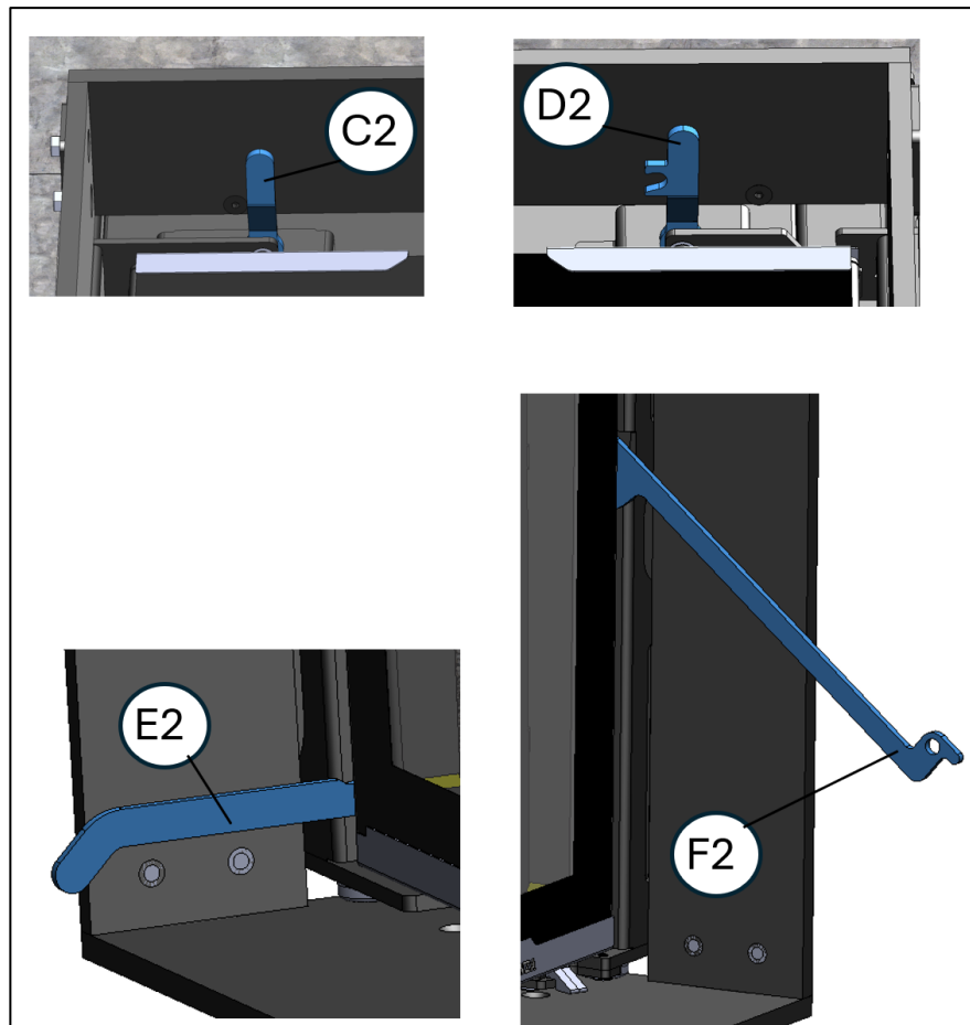
Figura nº29 - Elementos de funcionamiento del aparato IZARO 80-100 CLI
