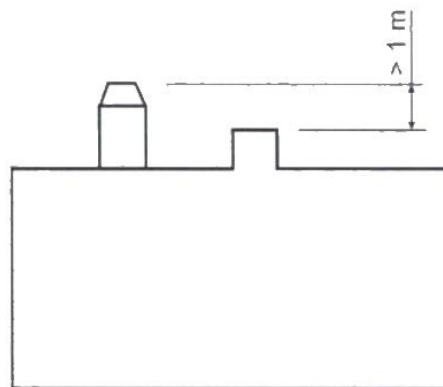
Figura nº23 - Distancias desde el remate hasta la cumbrera del tejado
