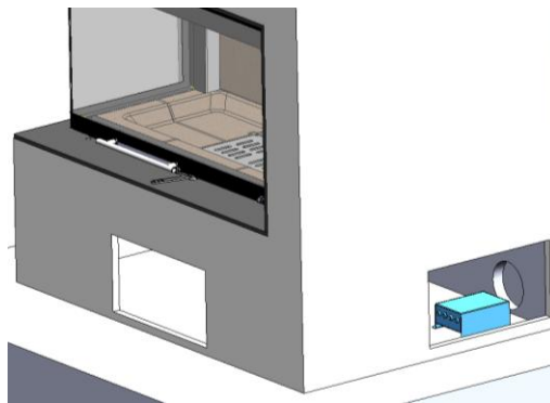
Figura n°21 - Posicionamiento del módulo de potencia frente a la rejilla de ventilación lateral
