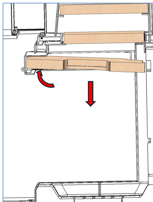
Figura n°33 - Desmontaje del deflector inferior izquierdo (lado cristal lateral)
