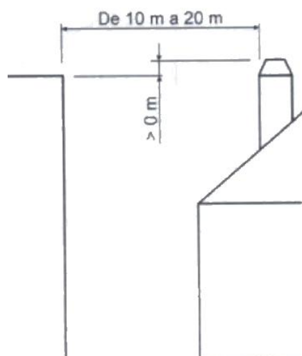
Figura n°25 - Distancias desde el remate hasta objetos entre 10 y 20m
