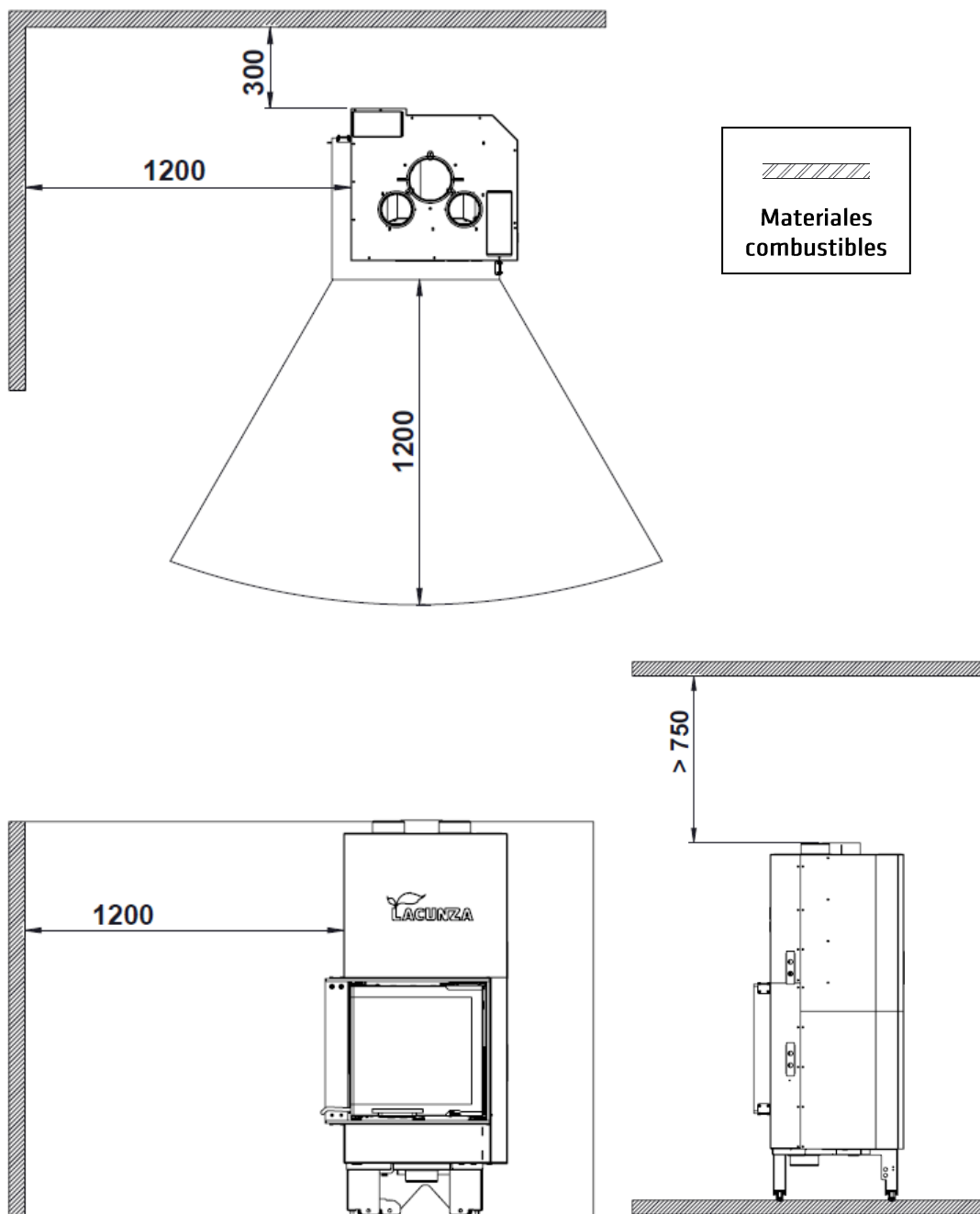
Figura nº3 - Distancias de seguridad Izaro 60/STAR CLI
