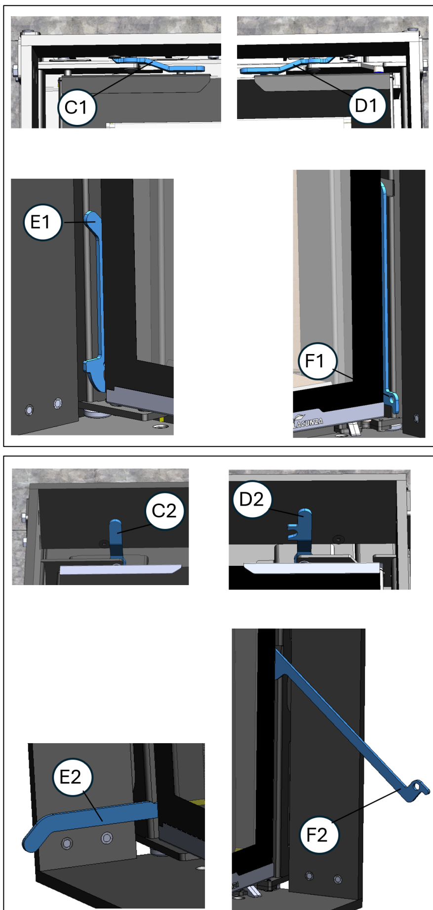
Figura nº27 - Elementos de funcionamiento del aparato IZARO 60 CLI
