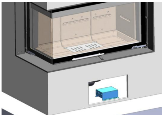
Figura n°20 - Posicionamiento del módulo de potencia frente a la rejilla de ventilación frontal
