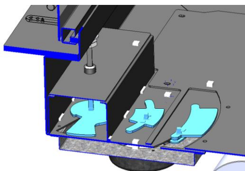
Figura n°45 - Acceso a Registros
