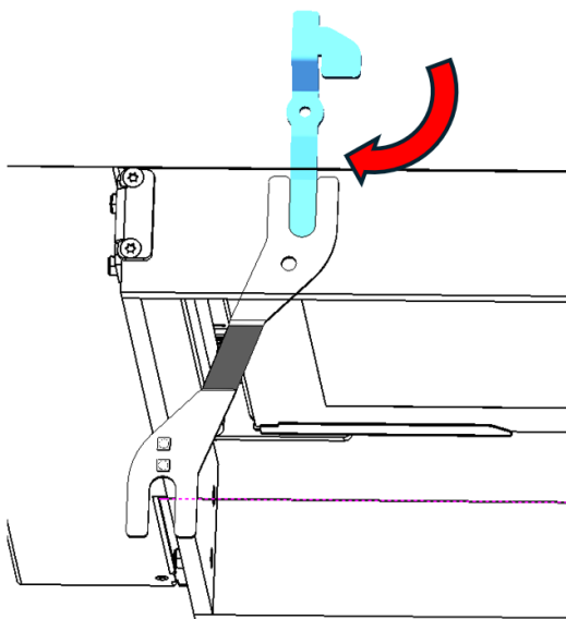
Figura n°39 - Girar la palanca superior-izq en el sentido de agujas reloj 90°
