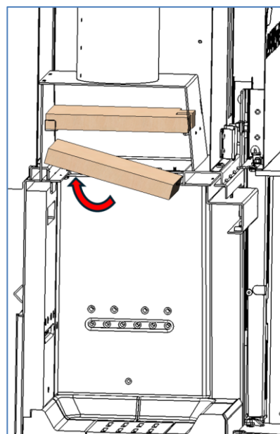
Figura n°34 - Desmontaje del deflector medio Izaro 60 CLI
