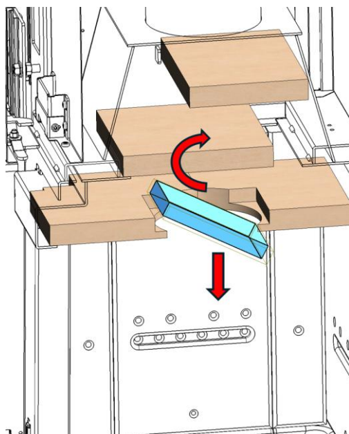
Figura n°31 - Desmontaje catalizador
