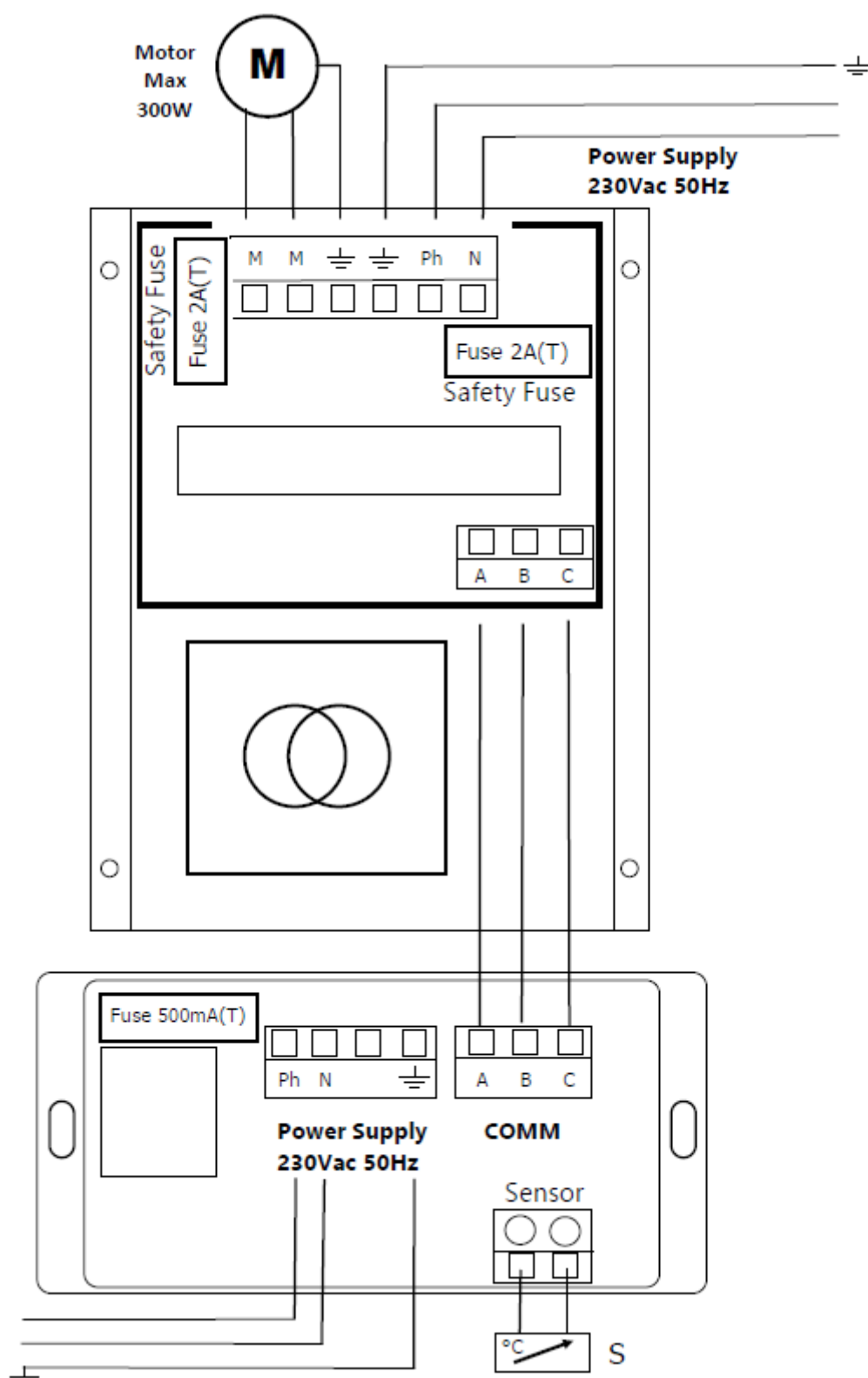
Figura n°18 - Conexiones a realizar en controlador y el módulo de potencia de la Iزارو C/V
