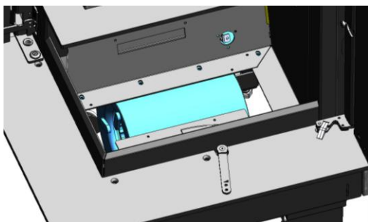
Figura n°44 - Acceso a la turbina a través del interior del hogar
