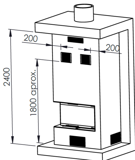
Figura nº8 - Esquema exterior del cerramiento
