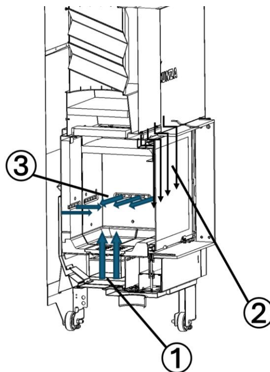
Figura n°28 - Entradas de aire de combustión
