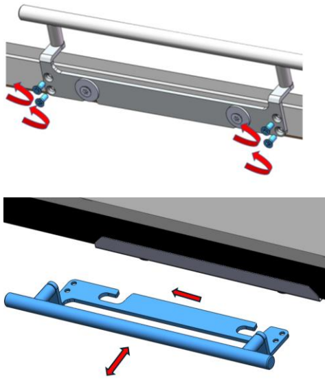
Figura n°42 - Extracción de tornillos y uso como mano fría de manilla.
