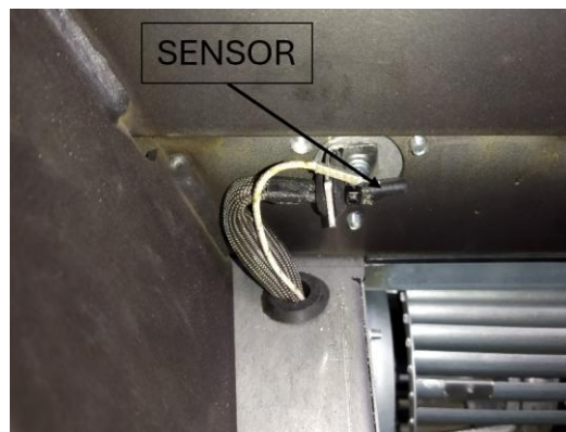
Figura n°22 - Posición de la sonda de temperatura (SENSOR) en la salida de aire de la turbina
