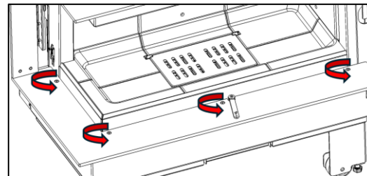
Figura nº15 - Destornillar los 8 tornillos, 4 superiores y 4 inferiores que amarran el marco exterior
