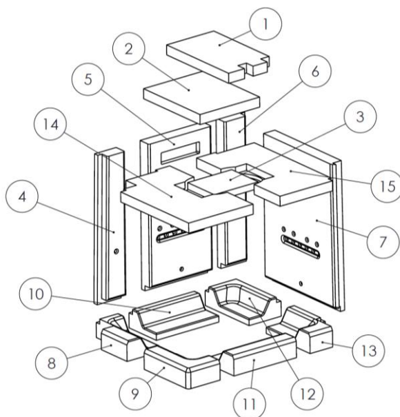
Figura nº47 - Despiece hogar vermi IZARO 60 CLI
