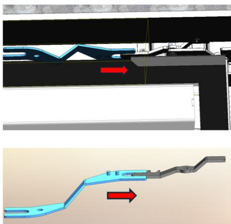
Figura n°37 - Introducir el útil manipulación en palanca giratoria superior dcha.
