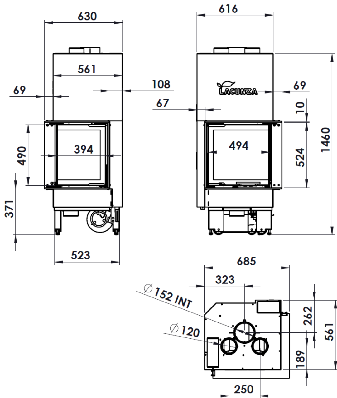
Figura nº2 - Dimensiones en mm del aparato IZARO 60/STAR CLD
