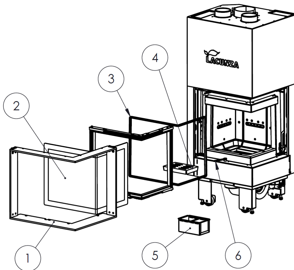
Figura n°48 - Despiece Izaro 60 CLD
