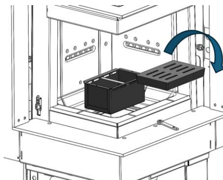
a- Retire la parrilla (14) y el cajetín cenicero (15).
