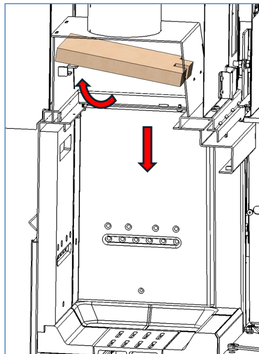
Figura n°35 - Desmontaje del deflector superior Izaro 60 CLI
