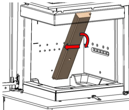
f- Retire la placa trasera derecha (6) desplazándola hacia el interior y dejándola caer hacia delante.
