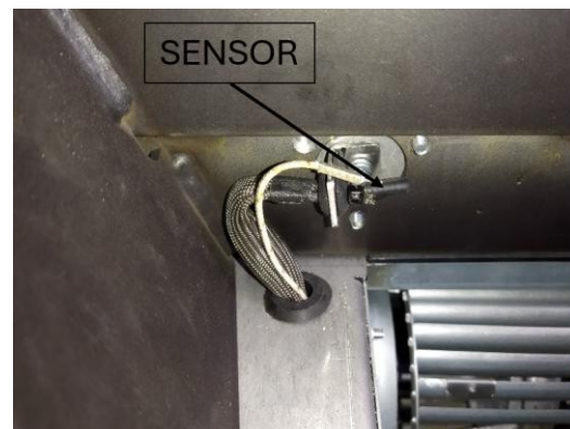
Figura n°22 - Posición de la sonda de temperatura (SENSOR) en la salida de aire de la turbina
