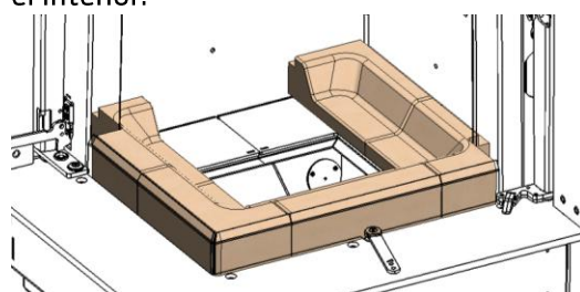
h- Retirar el resto de bases de vermiculita (8), (9), (11), (12), (13).
