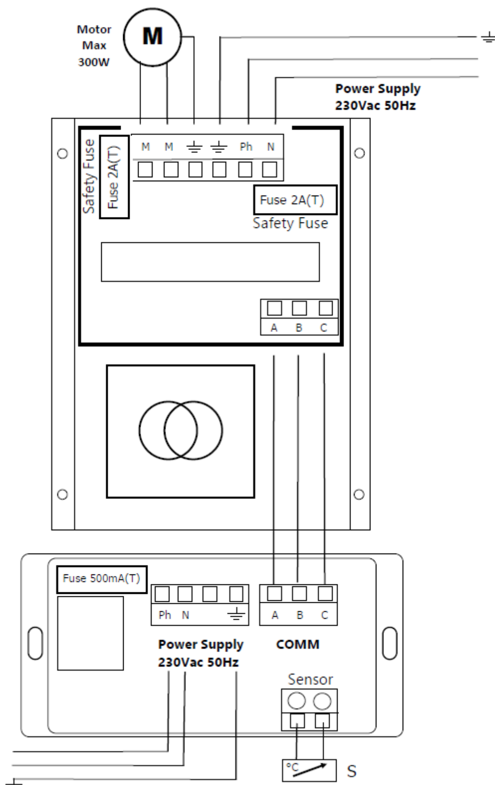
Figura nº18 - Conexiones a realizar en controlador y el módulo de potencia de la Iزارو C/V
