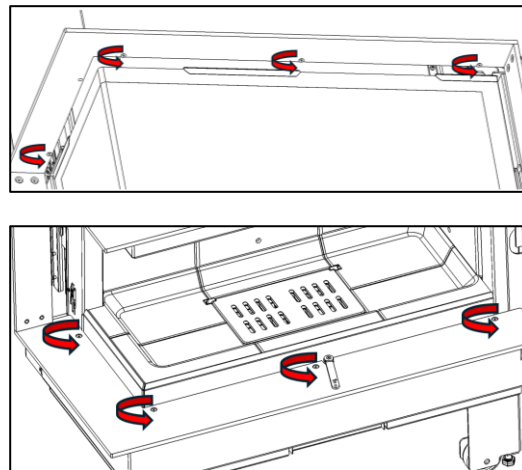
Figura n°15 - Destornillar los 8 tornillos, 4 superiores y 4 inferiores que amarran el marco exterior
