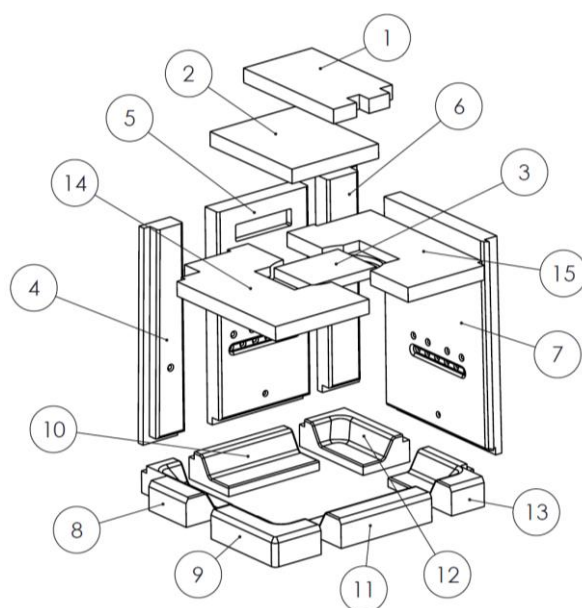
Figura n°47 - Despiece hogar vermi IZARO 60 CLI
