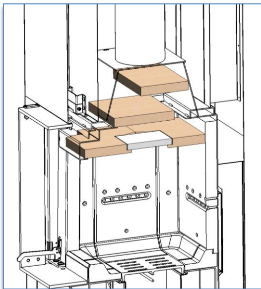
Figura n°30 - Vista de sección Izaro 60 CLI con los 3 deflectores colocados
