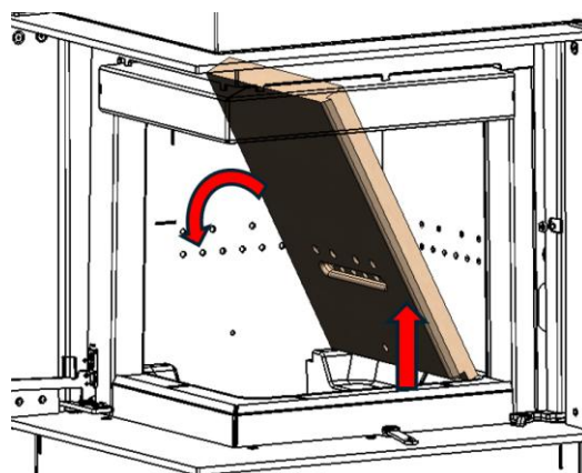
g- Retire la placa trasera lateral subiéndola y después dejándola caer hacia el interior.
