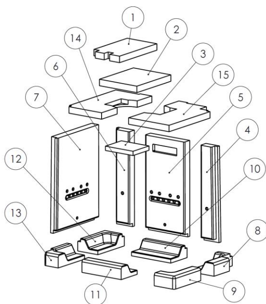
Figura n°49 - Despiece hogar vermi IZARO 60 CLD
