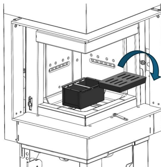
Figura n°29 - Retirada del cajón cenicero
