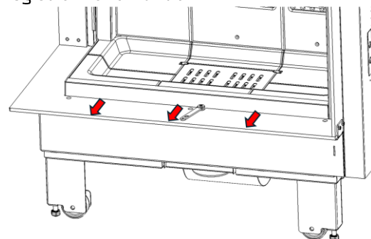
Figura n°16 - Extracción del marco exterior
