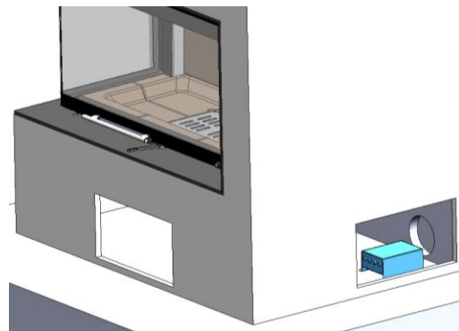
Figura n°21 - Posicionamiento del módulo de potencia frente a la rejilla de ventilación lateral
