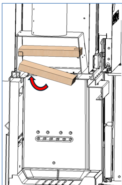
Figura n°34 - Desmontaje del deflector medio Izaro 60 CLI
