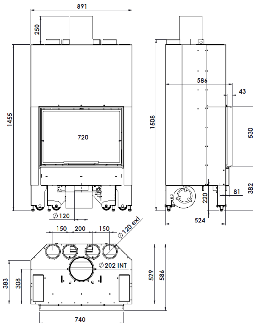
Figura n o 1 - Dimensiones en mm del aparato ITACA 80 eco
