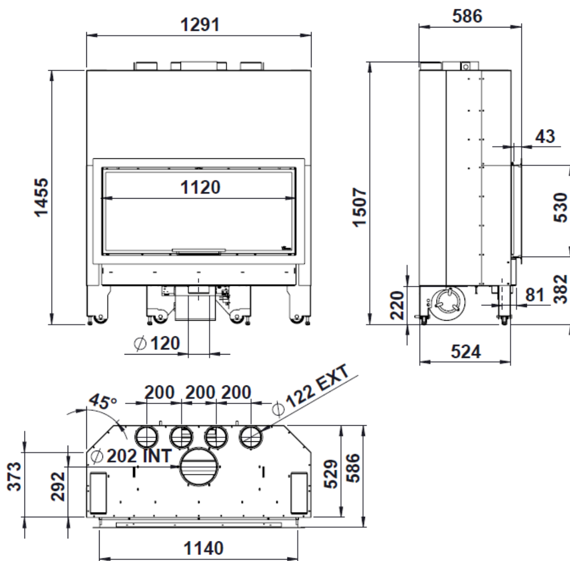
Figura nº3 - Dimensiones en mm Itaca 120 eco
