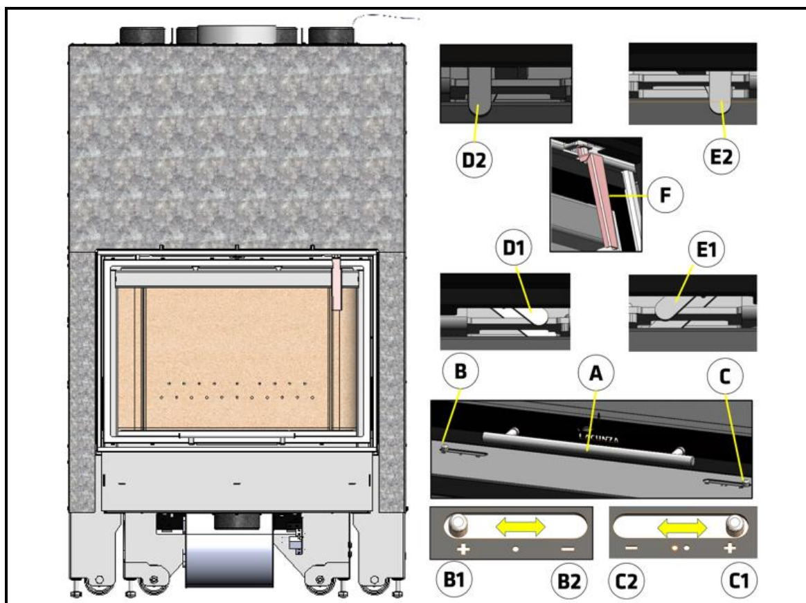
Figura nº26 - Elementos de funcionamiento del aparato
