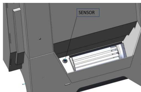
Figura nº21 - Posición de la sonda de temperatura (SENSOR) en la salida de aire de la turbina
