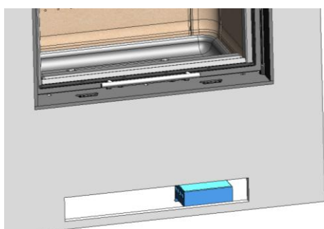
Figura nº19 - Posicionamiento del módulo de potencia frente a la rejilla de ventilación frontal
