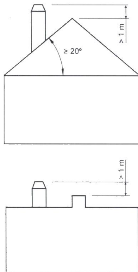
Figura nº22 - Distancias desde el remate hasta la cumbrera del tejado
