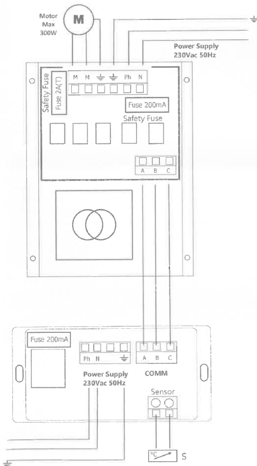
Figura nº17 - Conexiones a realizar en controlador y el módulo de potencia de la Itaca eco C/V
