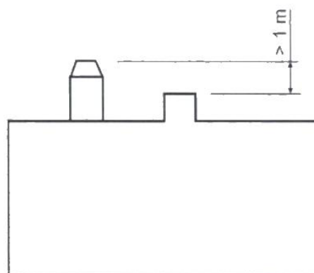
Figura nº18 - Distancias desde el remate hasta la cumbrera del tejado
