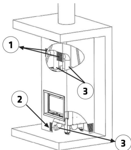
Figura nº8 - Imagen descriptiva de Opción B
