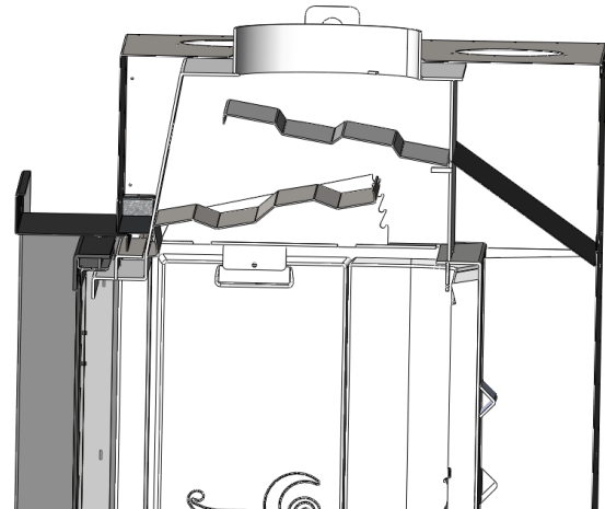
Figura nº18 - Vista de sección con los 2 deflectores colocados
