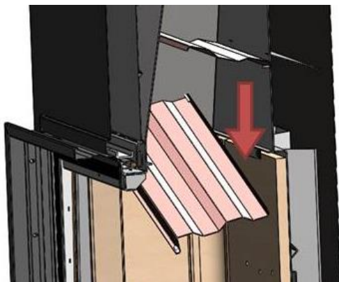
Figura nº20 - Desmontaje del deflector inferior Inca
