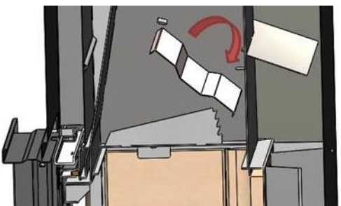
Figura nº21 - Desmontaje del deflector medio Inca
