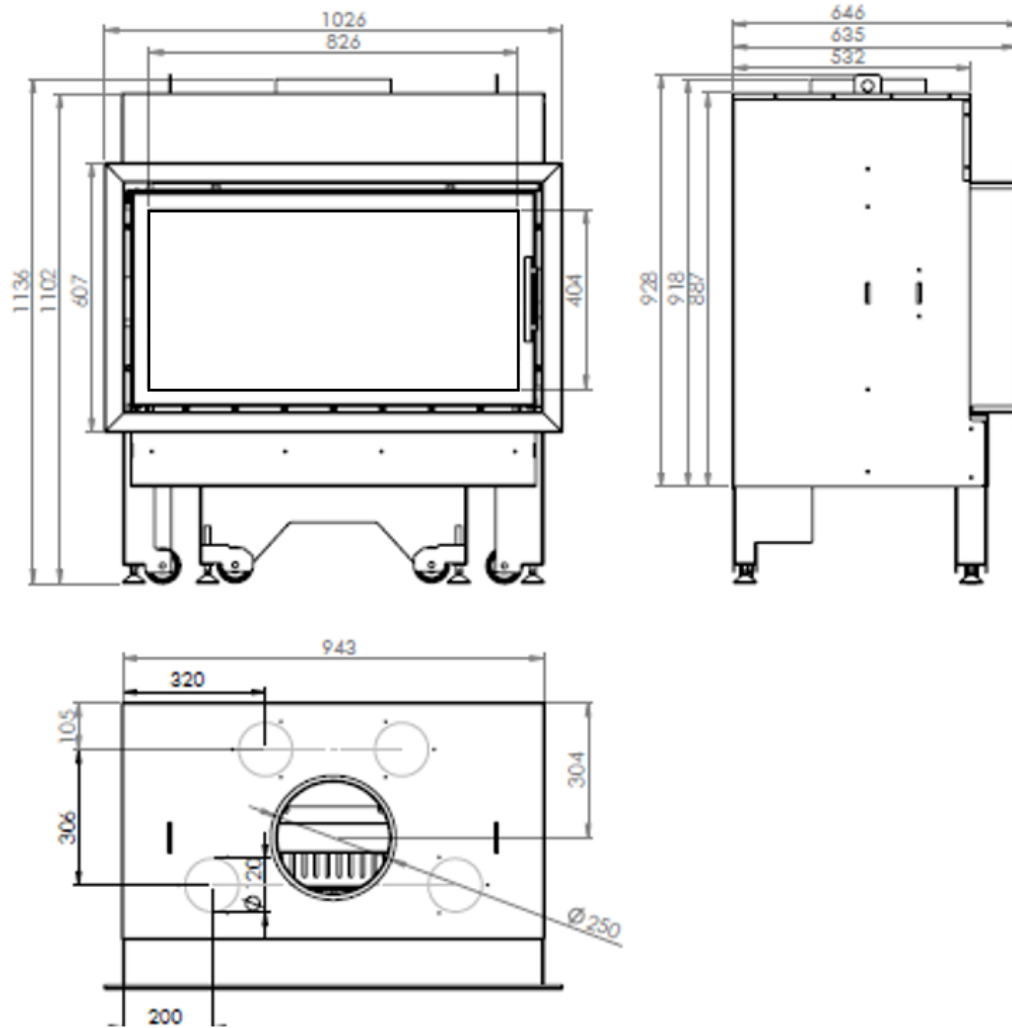
Figura nº2 - Dimensiones en mm aparato Inca 100
