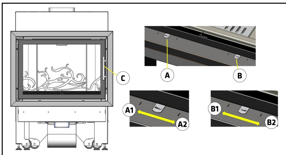
Figura nº17 - Elementos de funcionamiento del aparato
