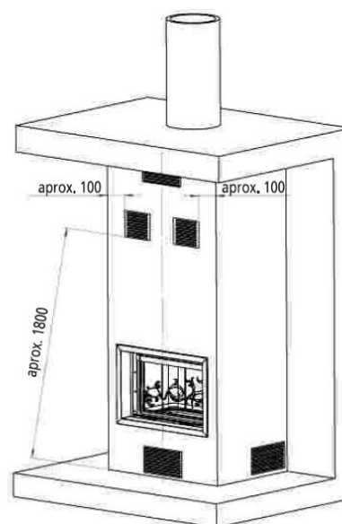
Figura nº7 - Esquema exterior del cerramiento
