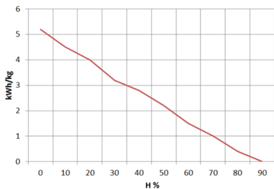
Figura nº11 - Relación entre humedad y poder calorífico de la leña.
