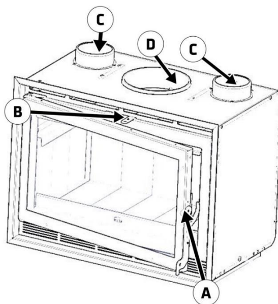
Figura nº12 - Elementos de funcionamiento del aparato
