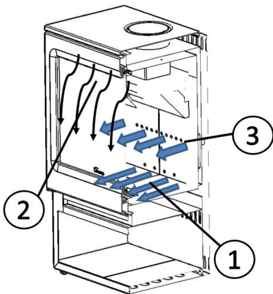
Figura n°11 - Entradas del aire de combustión
