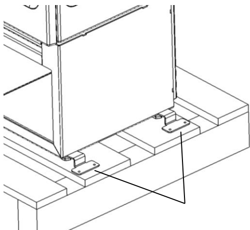
Figura nº4 - Detalle de las chapas que amarran las patas a la base de madera
