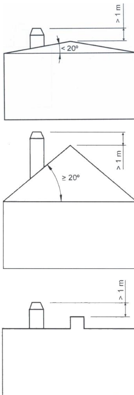
Figura nº6 - Distancias desde el remate hasta la cumbre del tejado
