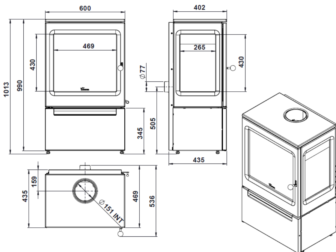
Figura nº1 - Dimensiones en mm de Garde
