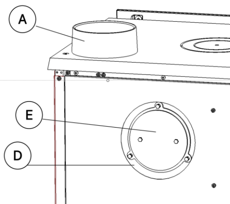
Figura nº7 - Situación final, apta para salida de humos superior.
