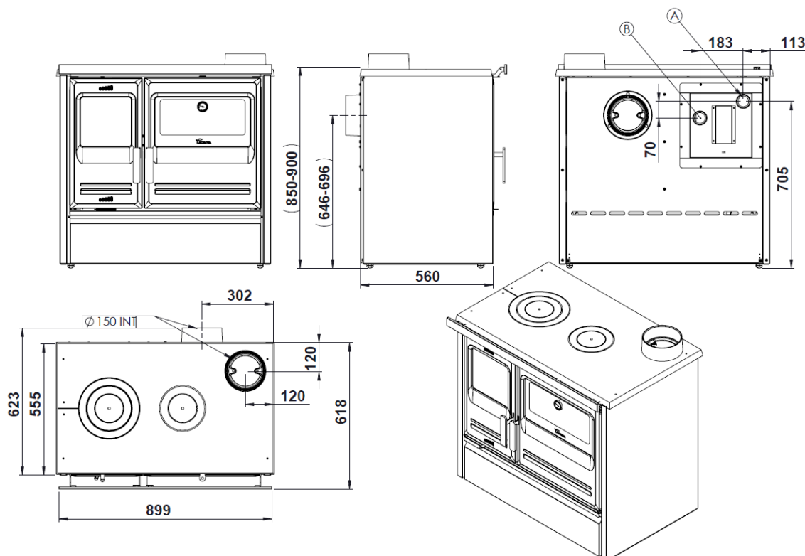
Figura nº1 - Dimensiones en mm del aparato ETNA 7T E
