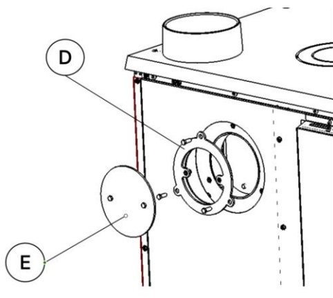
Figura nº6 - Colocamos el adaptador y la tapa.
