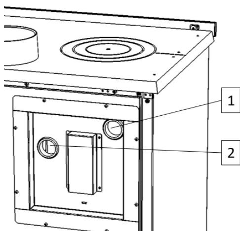
Figura n°12 - Racores de conexión en la paila
