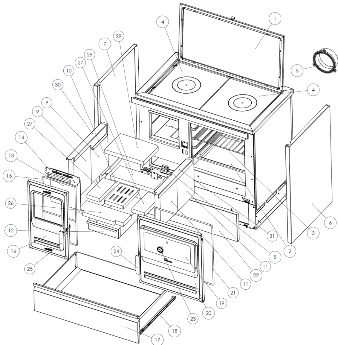
Figura nº24 - ETNA 7T
