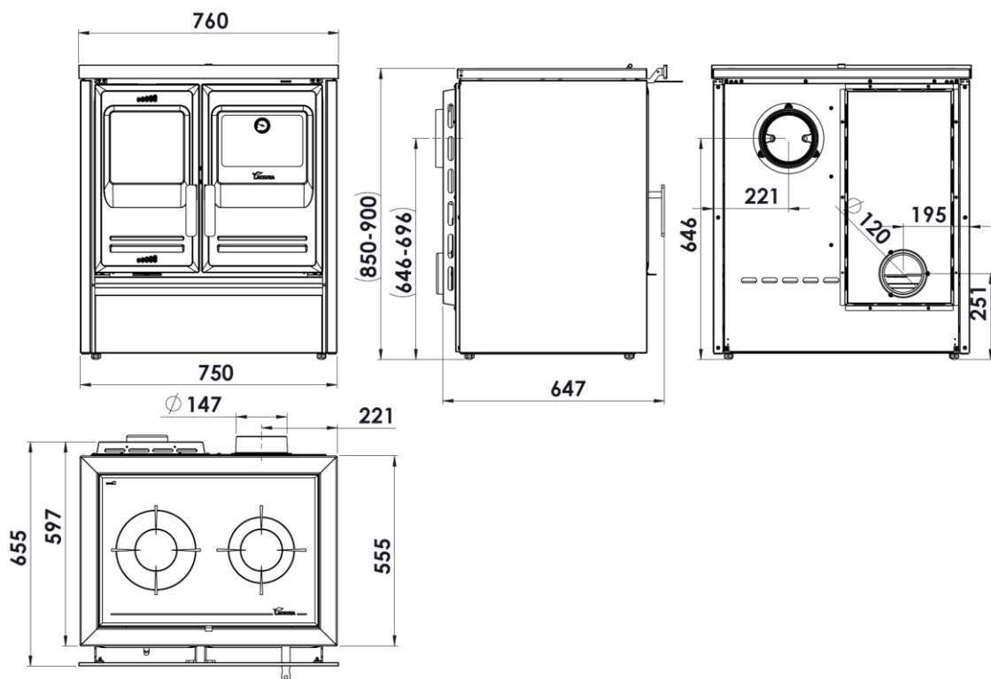
Figura n°2 - Dimensiones en mm del aparato ETNA 5T TOP
