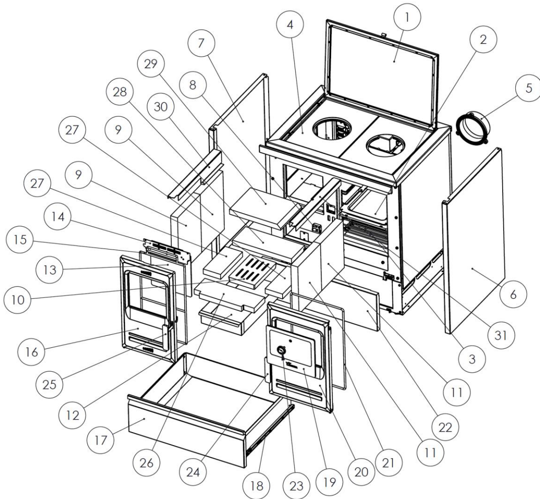
Figura nº23 - Etna 5T
