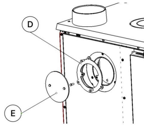
Figura nº9 - Colocamos el adaptador y la tapa.
