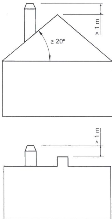
Figura nº12 - Distancias desde el remate hasta la cumbrera del tejado
