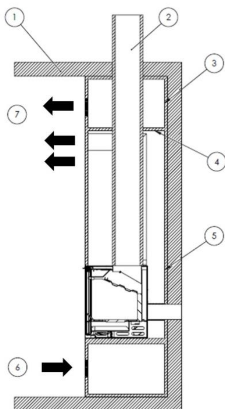
Figura n°3 - Esquema interior del cerramiento
