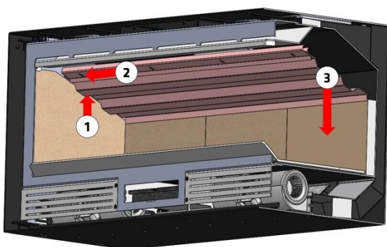
Figura n°18 - Desmontaje del deflector.
