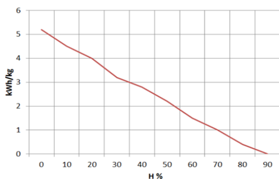
Figura n°14 - Relación entre humedad y poder calorífico de la leña.
