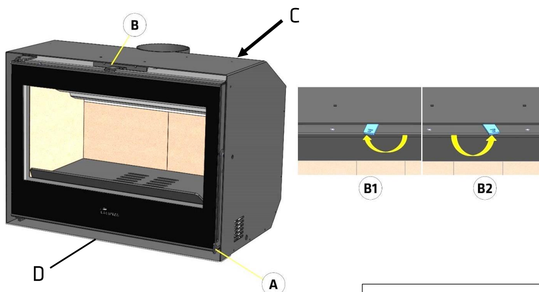
Figura n°15 - Elementos de funcionamiento del aparato
