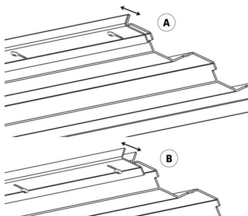
Figura n°17 - Diferentes posiciones del deflector inferior Chrome 700
